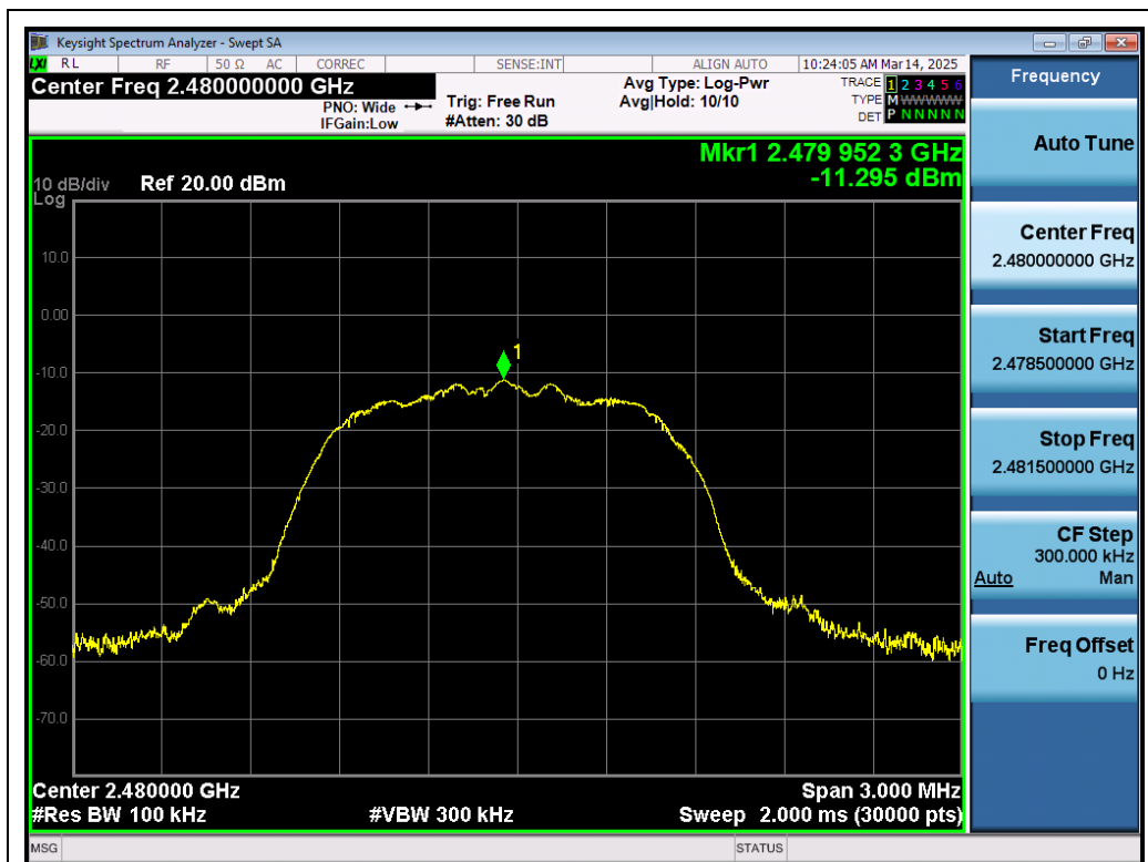
Test_Graph_EDR_ANT1_2480_3Mbps_Reference Level
