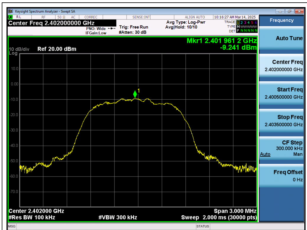
Test_Graph_EDR_ANT1_2402_3Mbps_Reference Level
