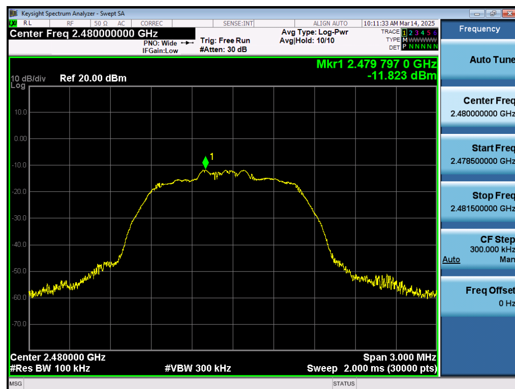
Test_Graph_EDR_ANT1_2480_2Mbps_Reference Level
