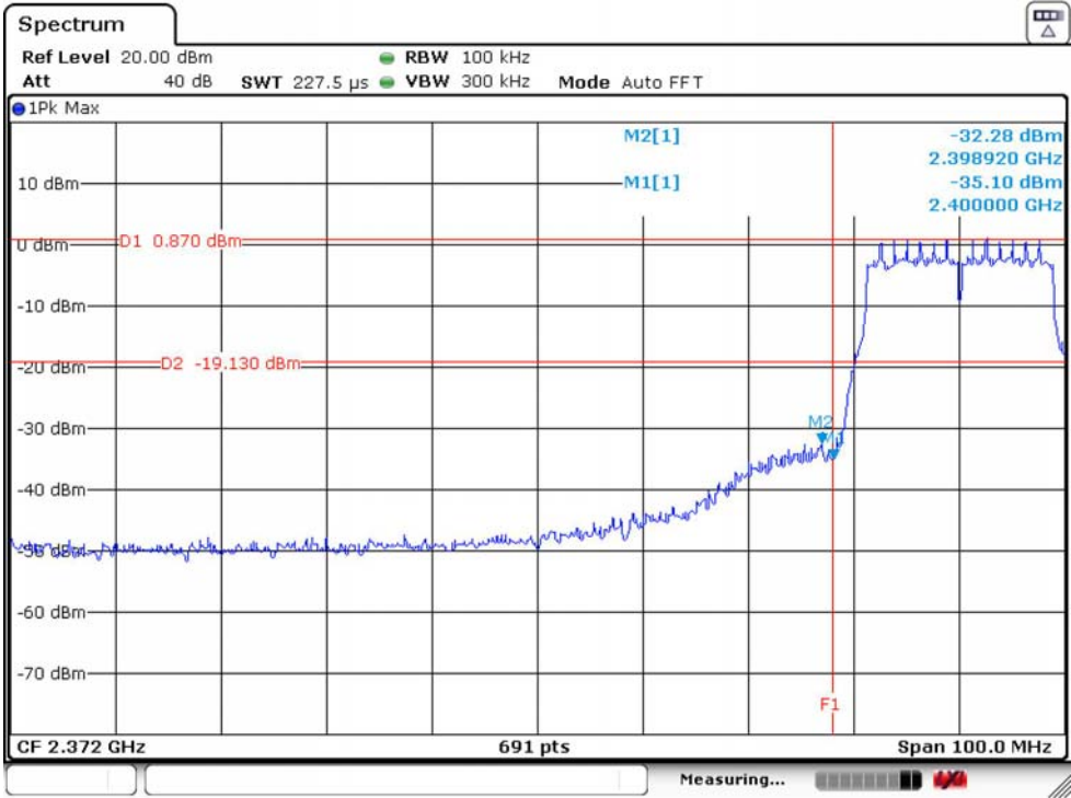
802.11n HT20 2412MHz_ANT 1
