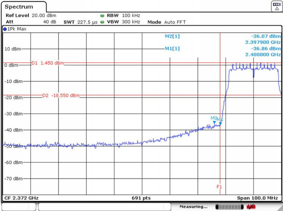
802.11n HT20 2412MHz_ANT 2
