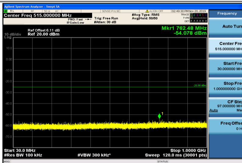
Band41-10MHz-QPSK-39700-1RB#0-30~1000MHz
