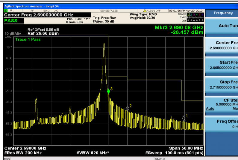
Band41-20MHz-QPSK-41490-1RB#99
