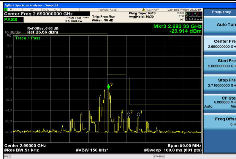
Band41-5MHz-16QAM-41565-1RB#24
