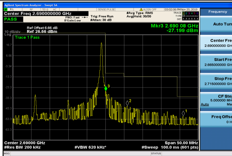
Band41-20MHz-16QAM-41490-1RB#99
