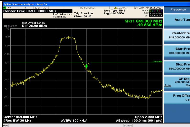
Band5-3MHz-QPSK-20635-1RB#14
