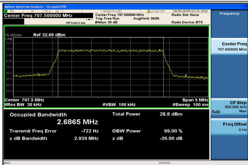
Band12-3MHz-QPSK-23095-15RB#0-2.6865
