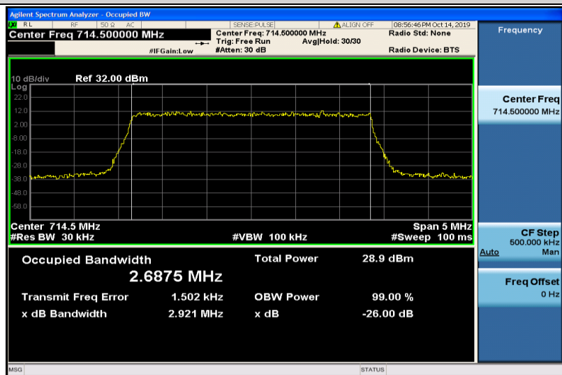
Band12-3MHz-QPSK-23165-15RB#0-2.6875
