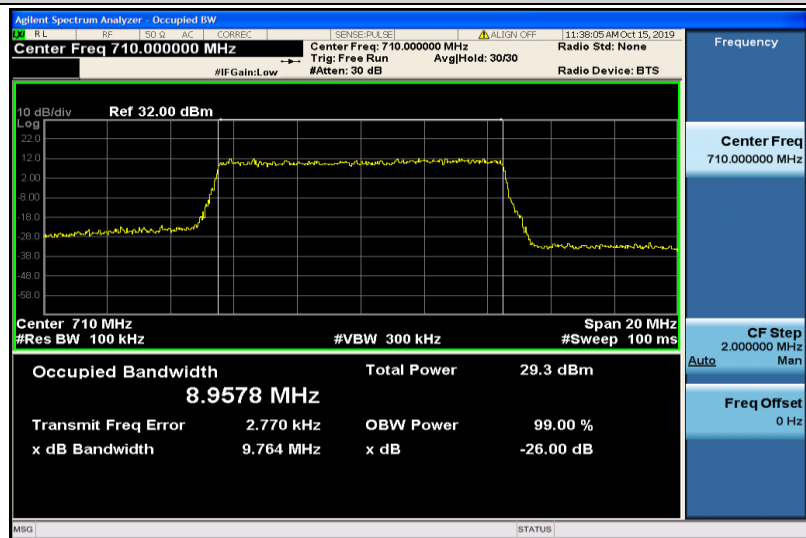
Band17-10MHz-QPSK-23790-50RB#0-8.9578
