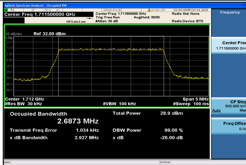
Band4-3MHz-QPSK-19965-15RB#0-2.6873
