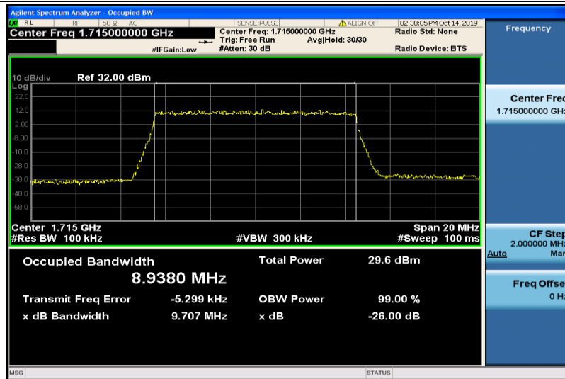
Band4-10MHz-QPSK-20000-50RB#0-8.9380
