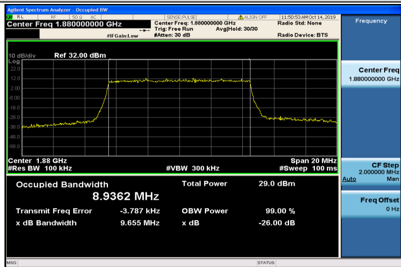
Band2-10MHz-QPSK-18900-50RB#0-8.9362
