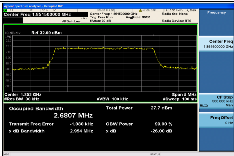
Band2-3MHz-16QAM-18615-15RB#0-2.6807
