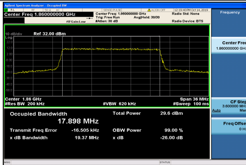
Band2-20MHz-QPSK-18700-100RB#0-17.898
