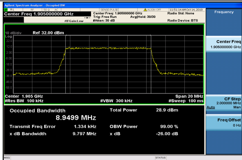
Band2-10MHz-QPSK-19150-50RB#0-8.9499
