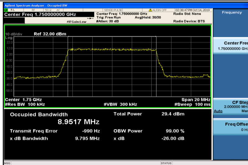
Band4-10MHz-QPSK-20350-50RB#0-8.9517
