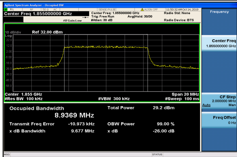
Band2-10MHz-QPSK-18650-50RB#0-8.9369
