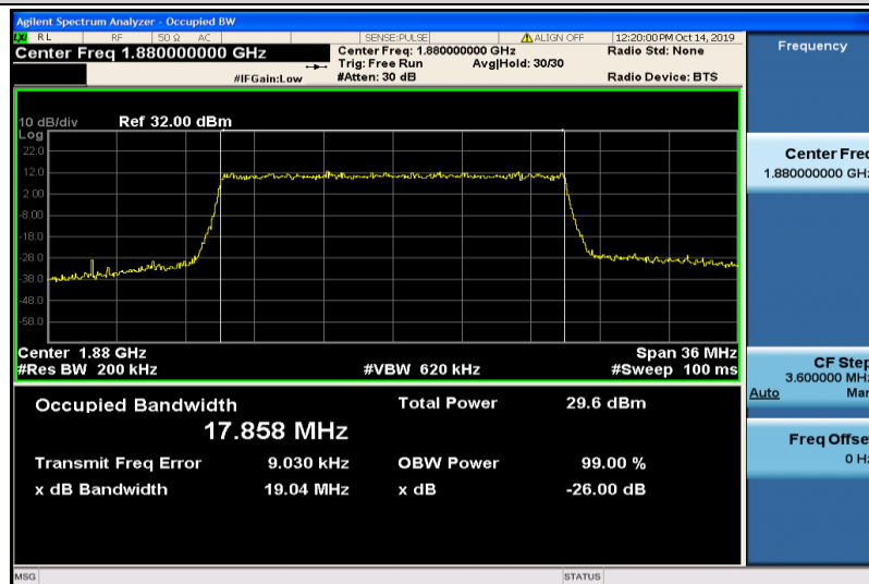
Band2-20MHz-QPSK-18900-100RB#0-17.858
