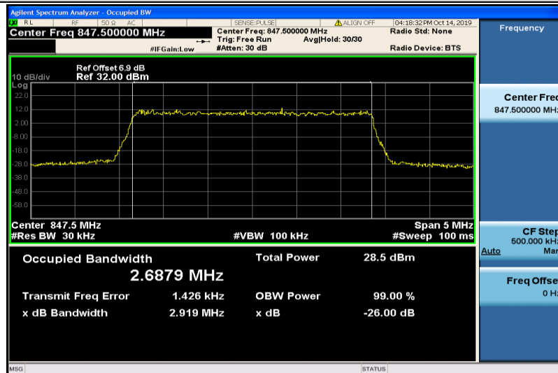
Band5-3MHz-QPSK-20635-15RB#0-2.6879
