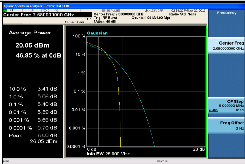
Band41-20MHz-16QAM-41490-1RB#0
