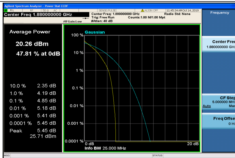
Band2-5MHz-QPSK-18900-25RB#0
