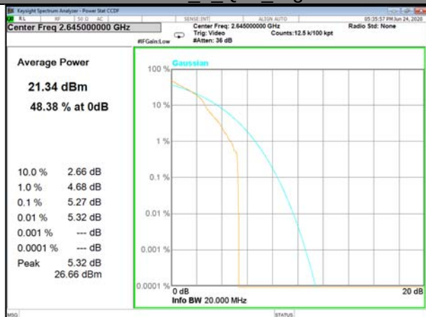
Band41_1_Q16_High
