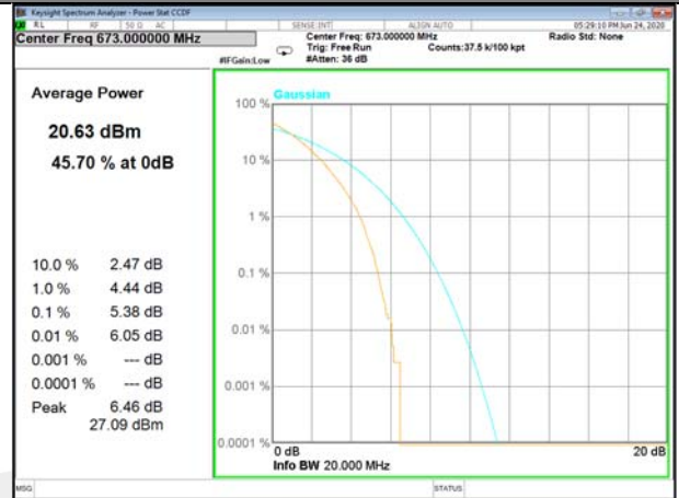
Band71_100_Q16_Low
