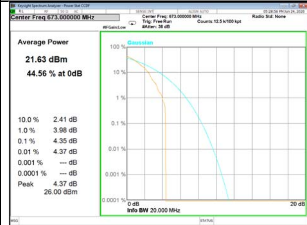
Band71_1_Q16_Low
