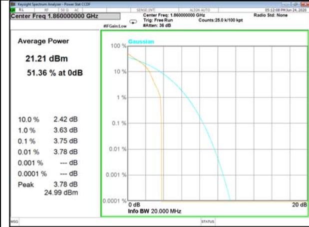
Band25_1_Q16_Low
