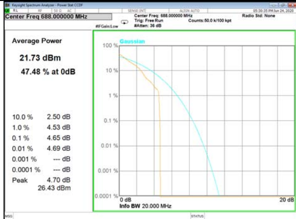
Band71_1_Q16_High
