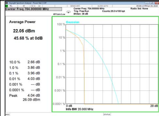
Band12_1_Q16_Low
