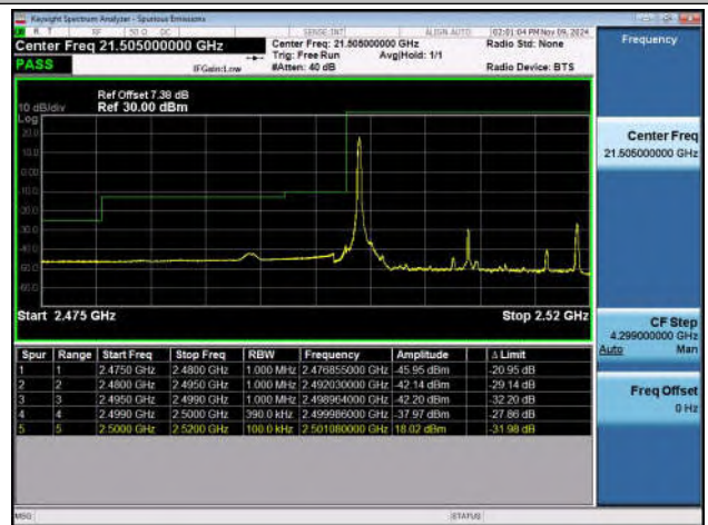
Band7_20MHz_QPSK_20850_1RB#0
