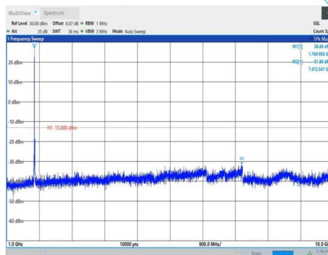
Band66-20MHz-QPSK-132572-1RB#0-Range2:1000~10000MHz
