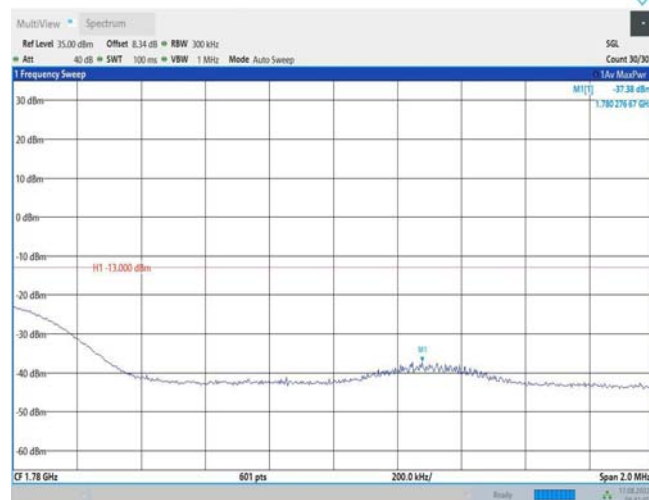
Band66-20MHz-QPSK-132572-1RB#99
