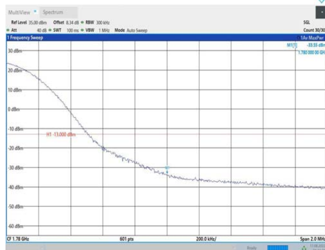
Band66-20MHz-QPSK-132572-100RB#0
