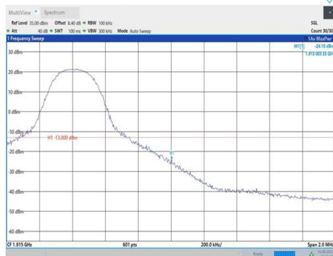
Band25-10MHz-QPSK-26640-50RB#0
