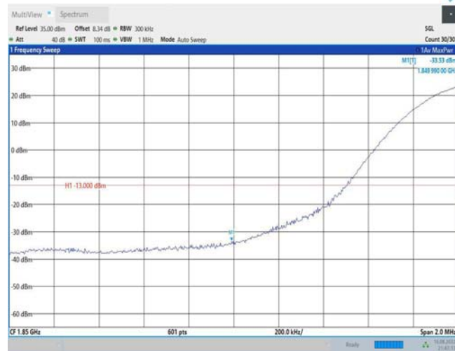
Band25-20MHz-QPSK-26140-1RB#99
