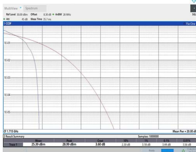
Band66-10MHz-QPSK-132022-50RB#0
