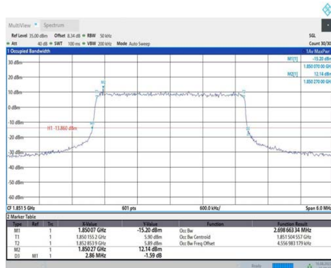
Band25-3MHz-QPSK-26365-15RB#0
