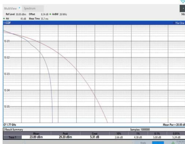
Band66-20MHz-QPSK-132572-100RB#0
