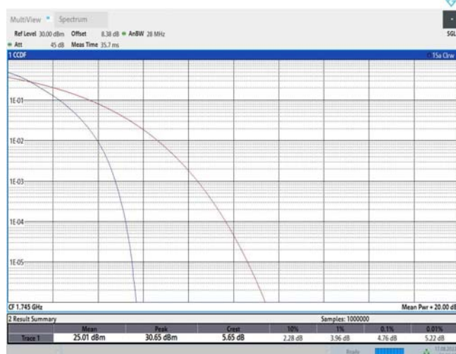
Band66-20MHz-QPSK-132572-1RB#0
