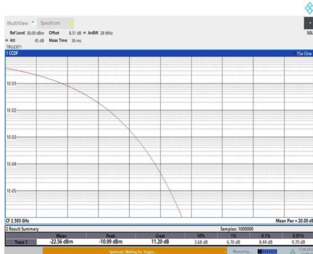
Band41-20MHz-QPSK-41490-1RB#0
