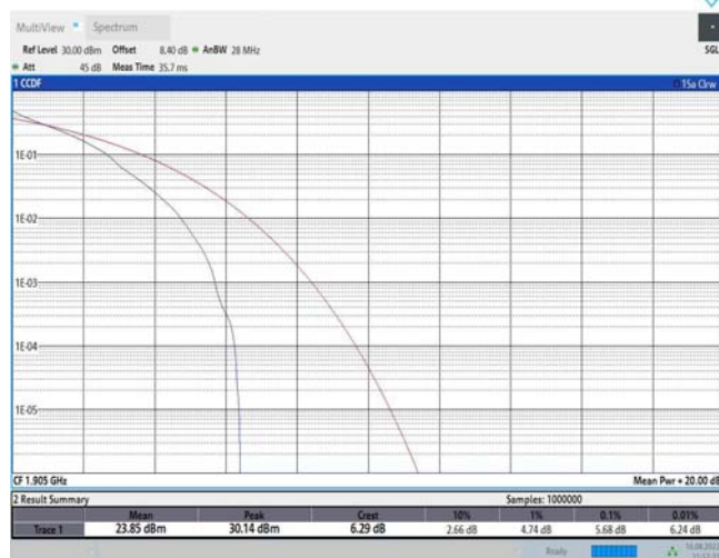
Band25-20MHz-QPSK-26590-100RB#0
