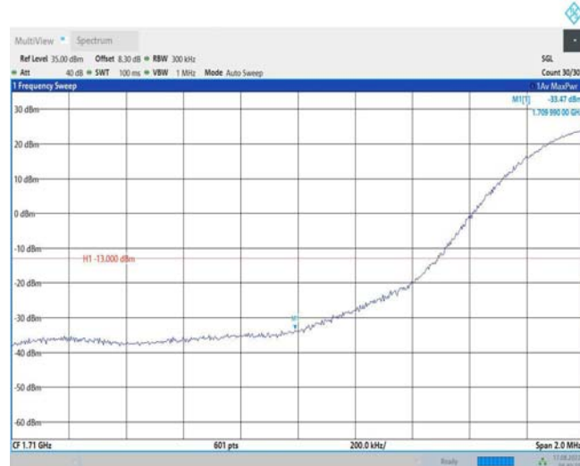
Band66-20MHz-QPSK-132072-1RB#99
