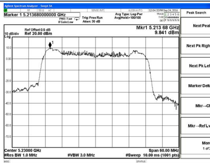
Chain 1-5230MHz
