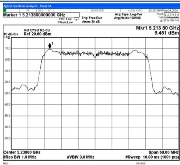
Chain 0-5230MHz
