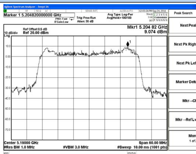
Chain 1-5190MHz
