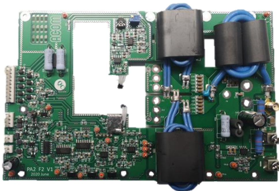
Figure 11 - PA2 F2 V1 top side
