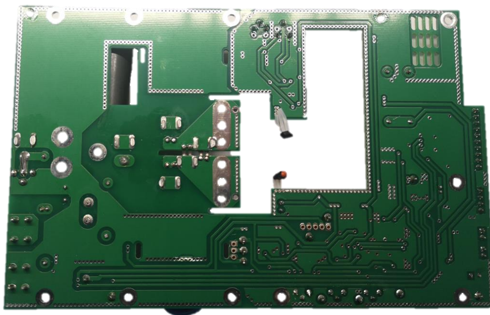
Figure 11 - PA2 F2 V1 top side
