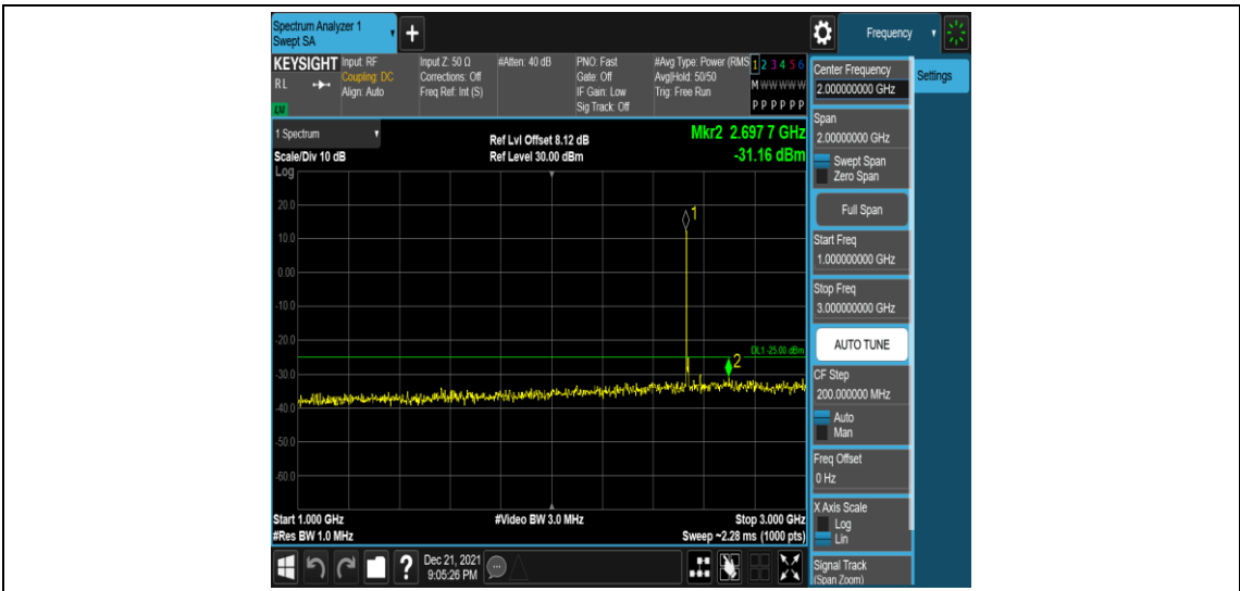
Band7-10MHz-QPSK-21100-1RB#0-Range4:1000~3000MHz
