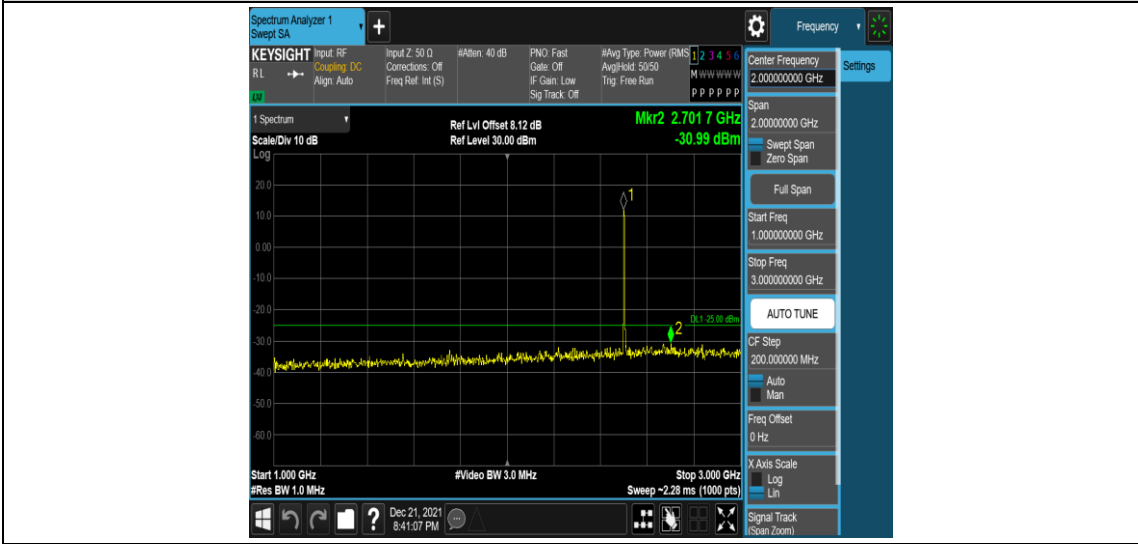
Band7-5MHz-QPSK-20775-1RB#0-Range4:1000~3000MHz
