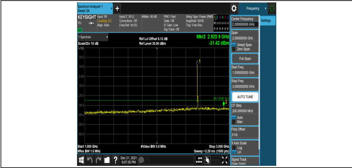
Band7-10MHz-QPSK-21400-1RB#0-Range4:1000~3000MHz
