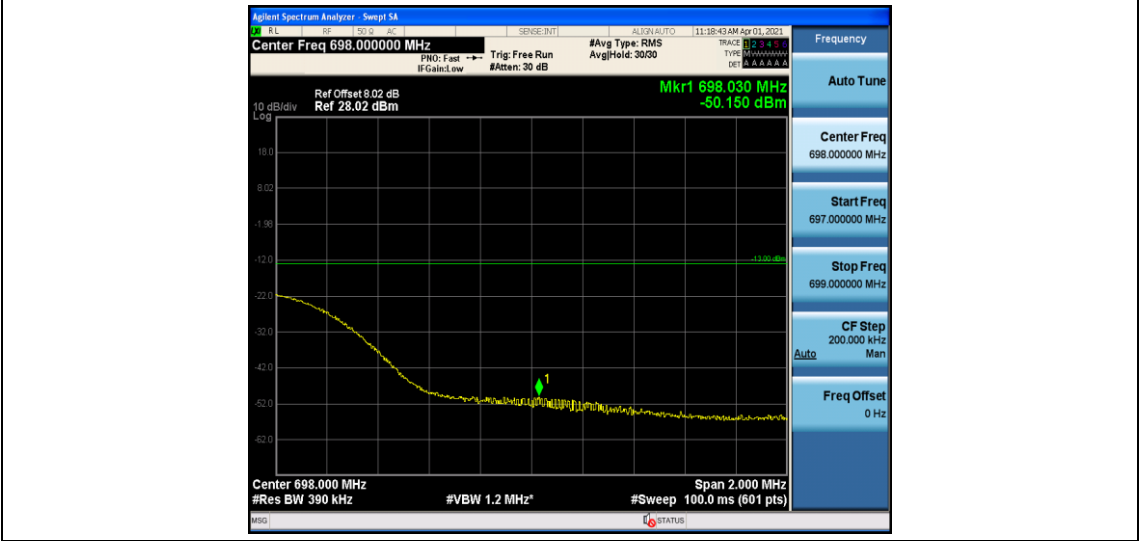
Band71_20MHz_QPSK_133372_1RB#99
