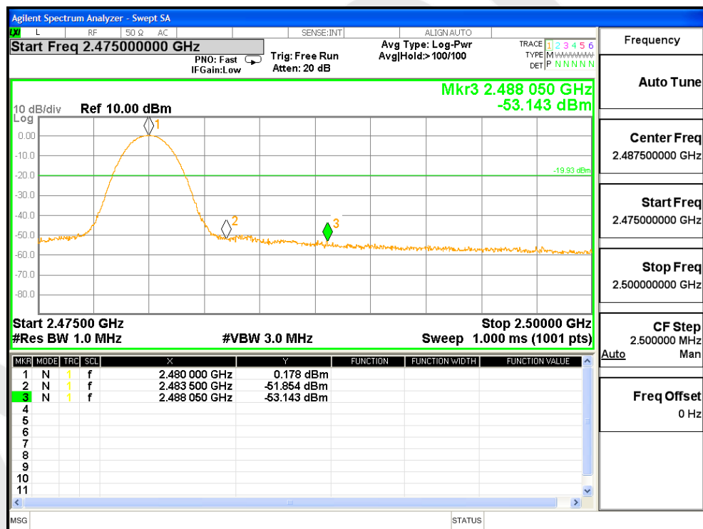
\pi/4 DQPSK mode -- Highest
