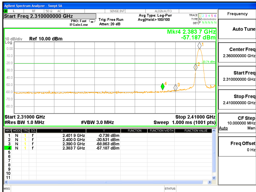
\pi/4 DQPSK mode -- Lowest
