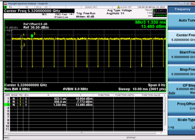
U-NII-2a,802.11n(HT20),5320MHz ,Ant0
