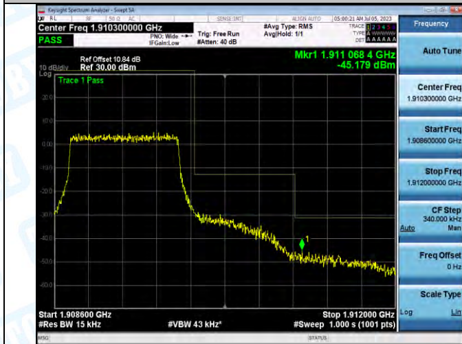
Band2_Band2_1.4MHz_QPSK_19193_6RB#0
