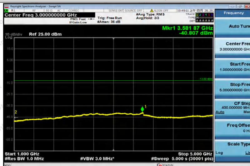
Band5-1.4MHz-QPSK-20407-1RB#0-Range2:1000~5000MHz
