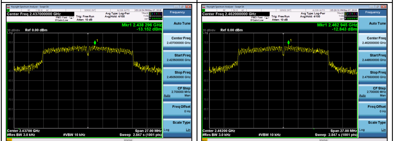
PSD - Mid CH 2437 - 802.11g
