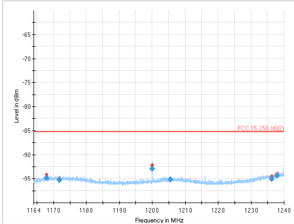
Plot 12: 1164 MHz to 1240 MHz (§15.250 (d)(2), RSS-210 K.3(b))
