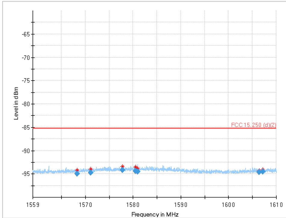
Plot 13: 1559 MHz to 1610 MHz (§15.250 (d)(2), RSS-210 K.3(b))
