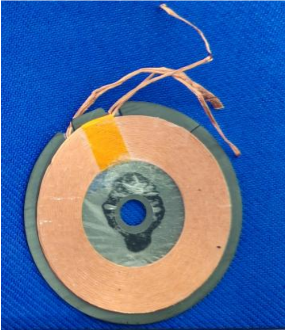
EUT Photo
