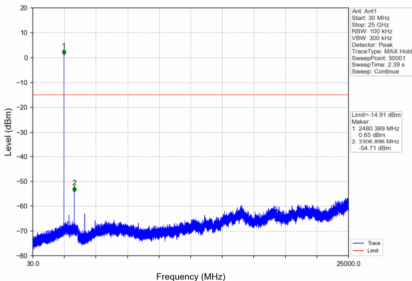
2M_HCH_2480MHz_DataRate=_Ant1_NTNV
