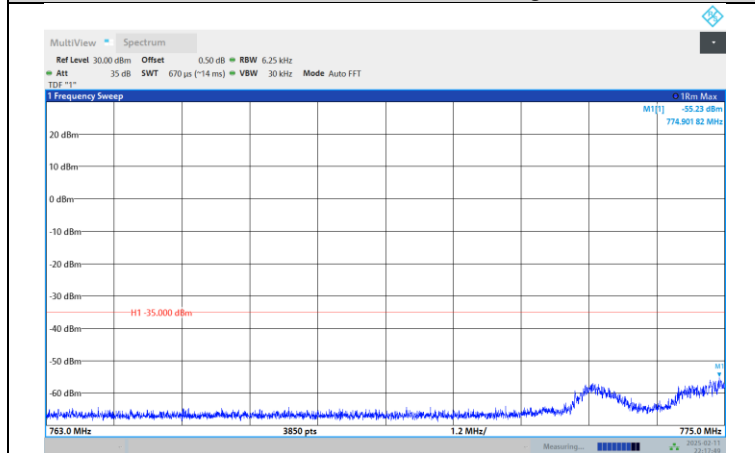
Band13-5MHz-QPSK-23230-1RB#0-Range:763~775MHz
