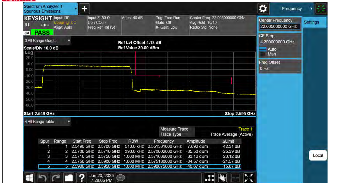
Band7-20MHz-QPSK-21350-1RB#99-PASS
