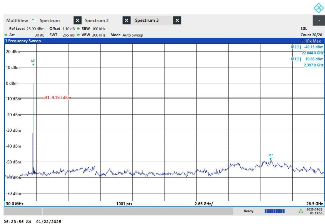
DH5_ANT7_2402_30~26500
