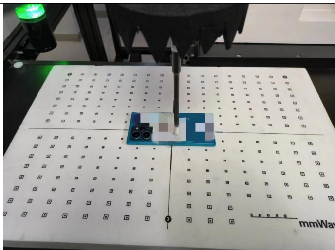
Back( \lambda/5=8.58\text{mm} )
