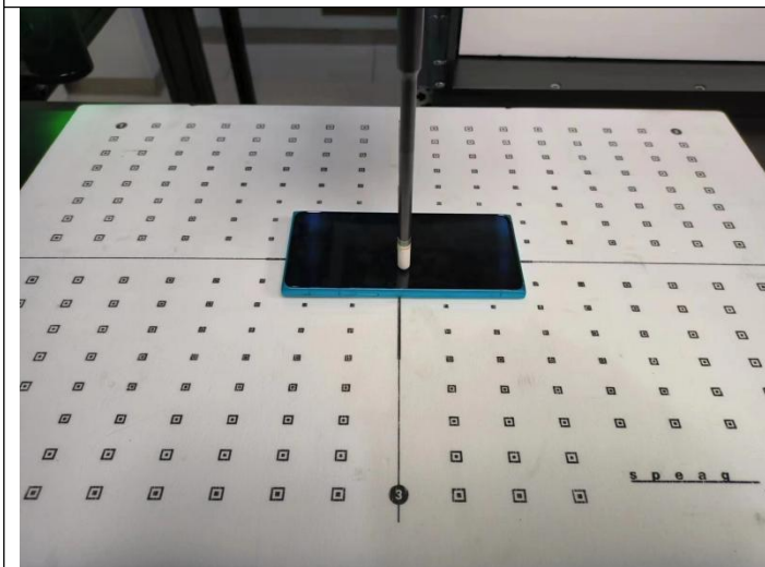
Front(2mm)
