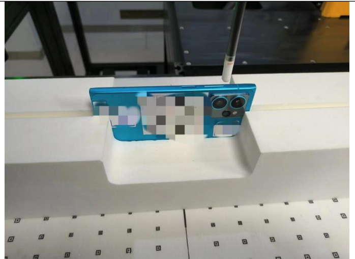
Right(2mm)
