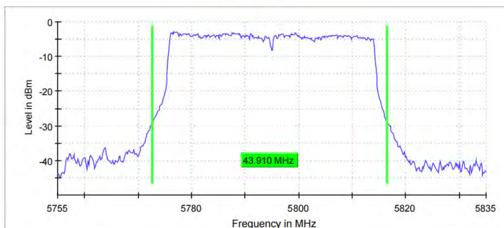
11AX40MIMO_Ant11_5795_484Tone_RU65
