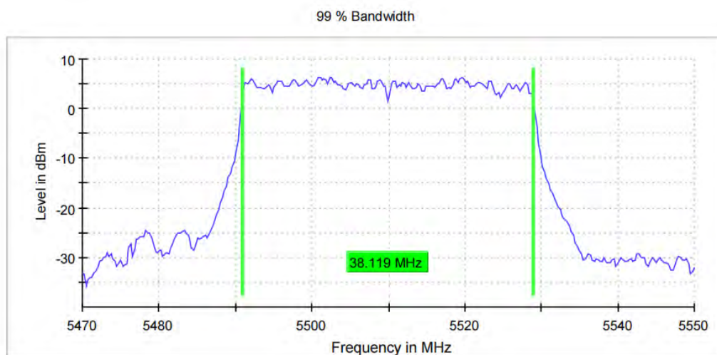
11AX40MIMO_Ant11_5510_484Tone_RU65
