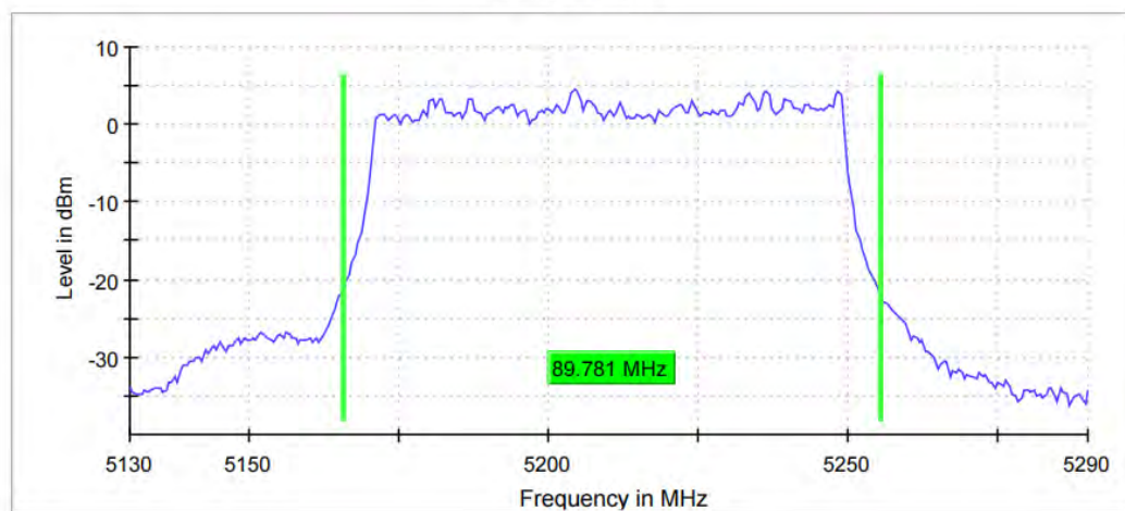
11AX80MIMO_Ant8_5210_996Tone_RU67
