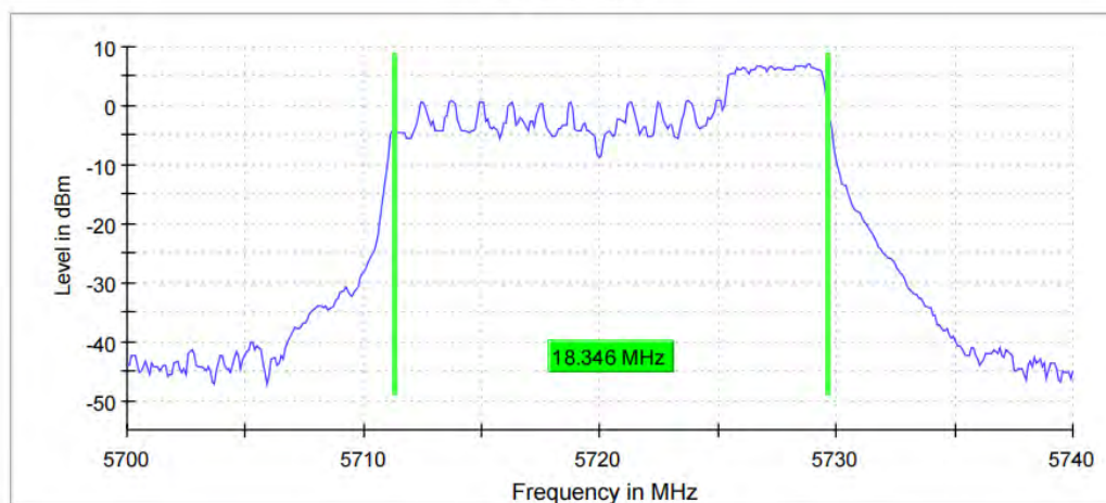
11AX20MIMO_Ant11_5720_106Tone_RU53
