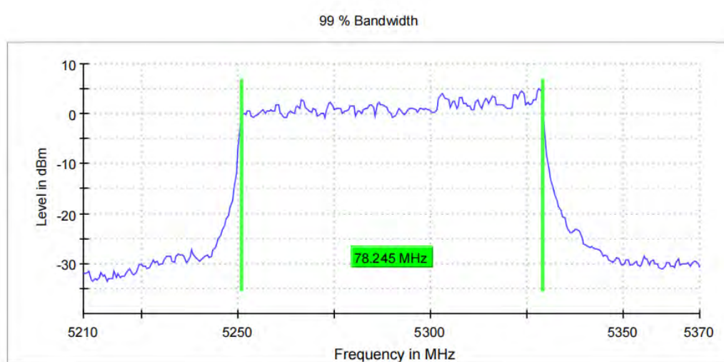
11AX80MIMO_Ant11_5290_996Tone_RU67
