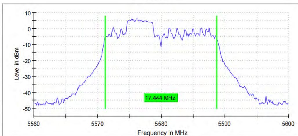
11AX20MIMO_Ant8_5580_106Tone_RU53
