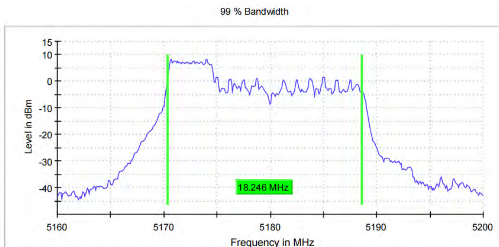
11AX20MIMO_Ant11_5180_106Tone_RU53
