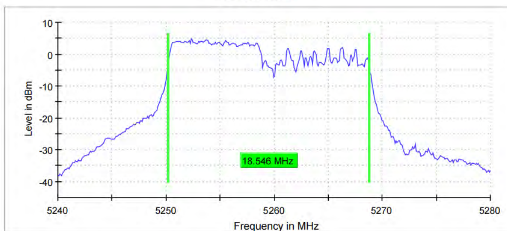
11AX20MIMO_Ant8_5260_242Tone_RU61
