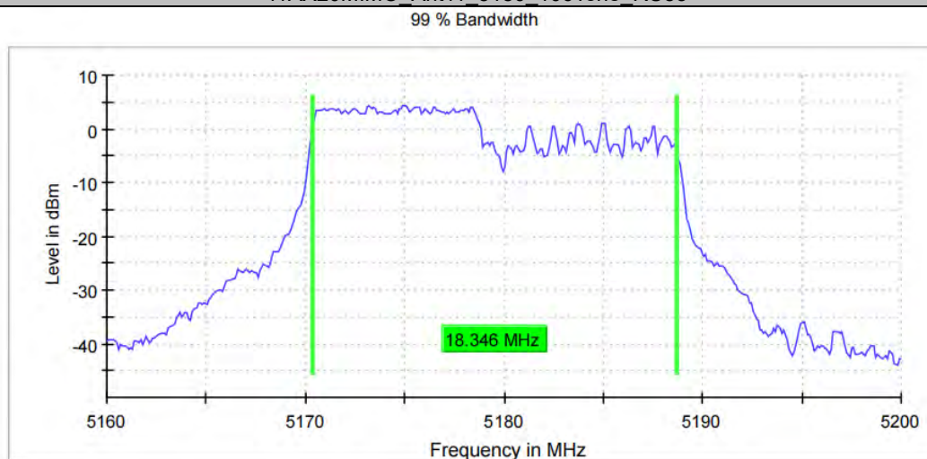
11AX20MIMO_Ant11_5180_106Tone_RU53
