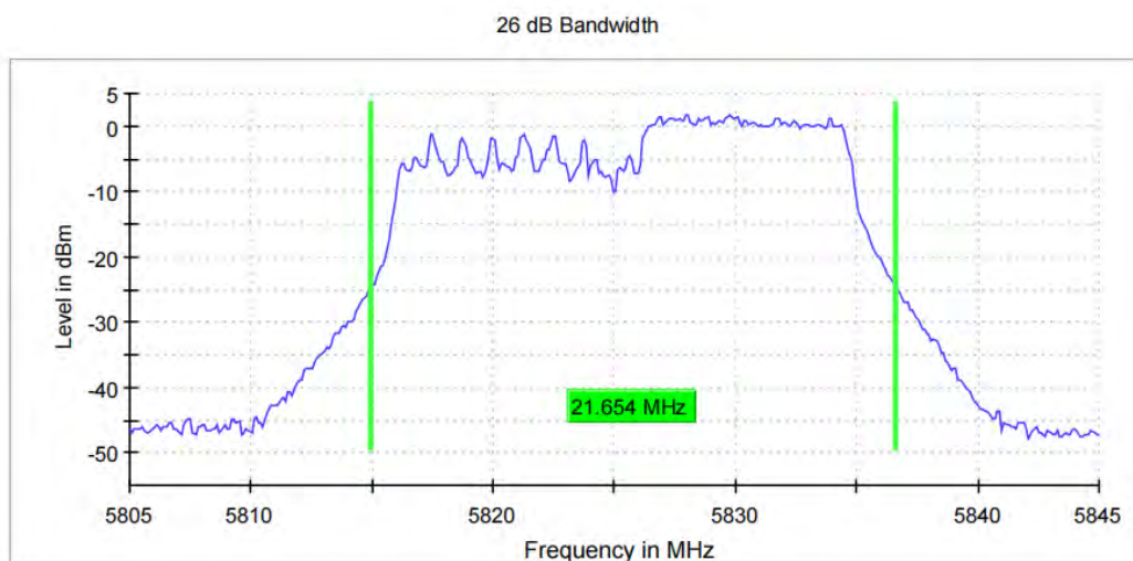
11AX20MIMO_Ant8_5825_106Tone_RU53
