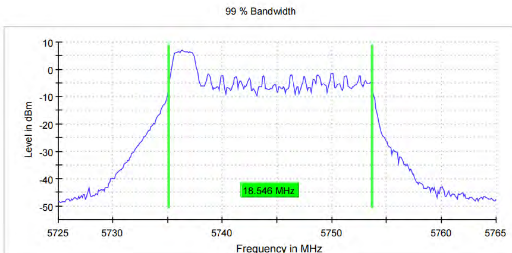
11AX20MIMO_Ant11_5745_26Tone_RU0
