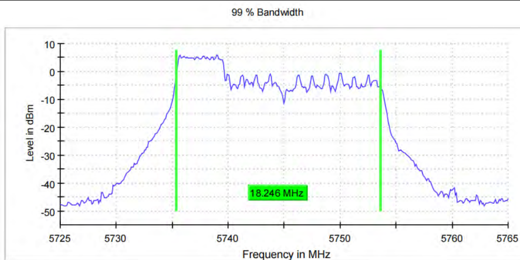
11AX20MIMO_Ant11_5745_52Tone_RU37
