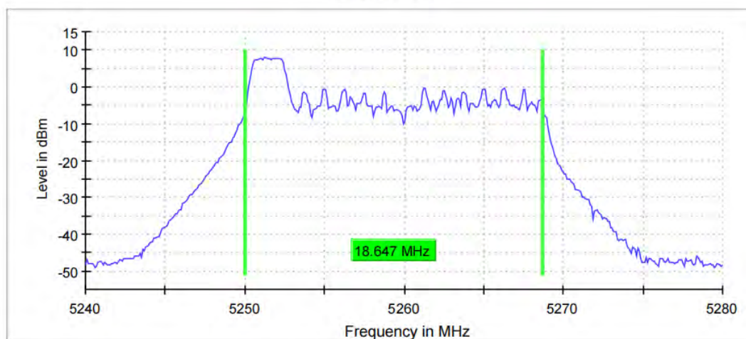
11AX20MIMO_Ant8_5260_26Tone_RU0
