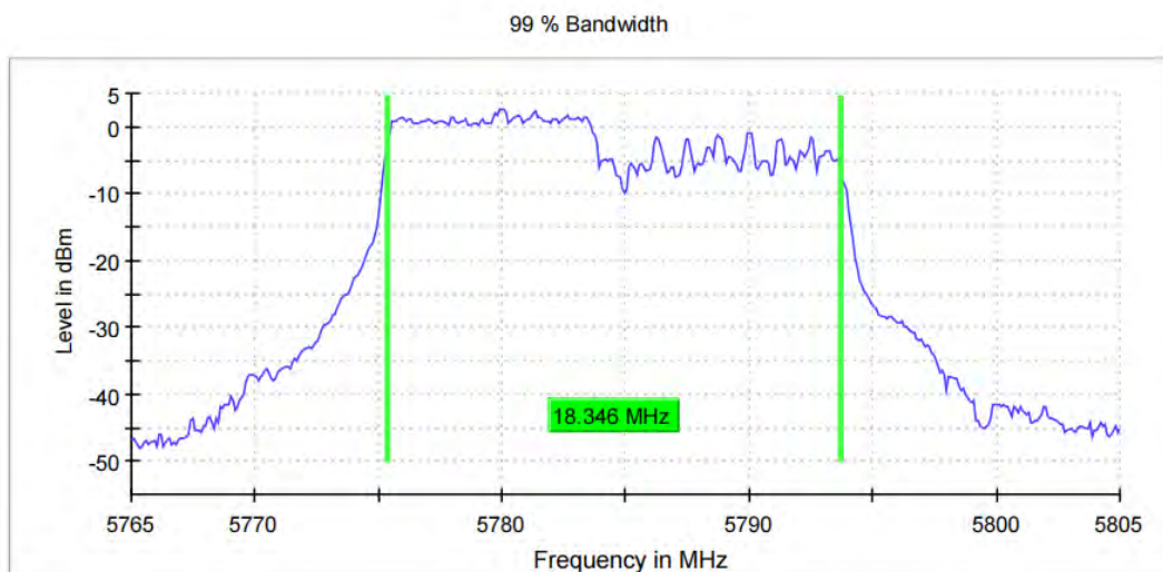
11AX20MIMO_Ant11_5785_242Tone_RU61
