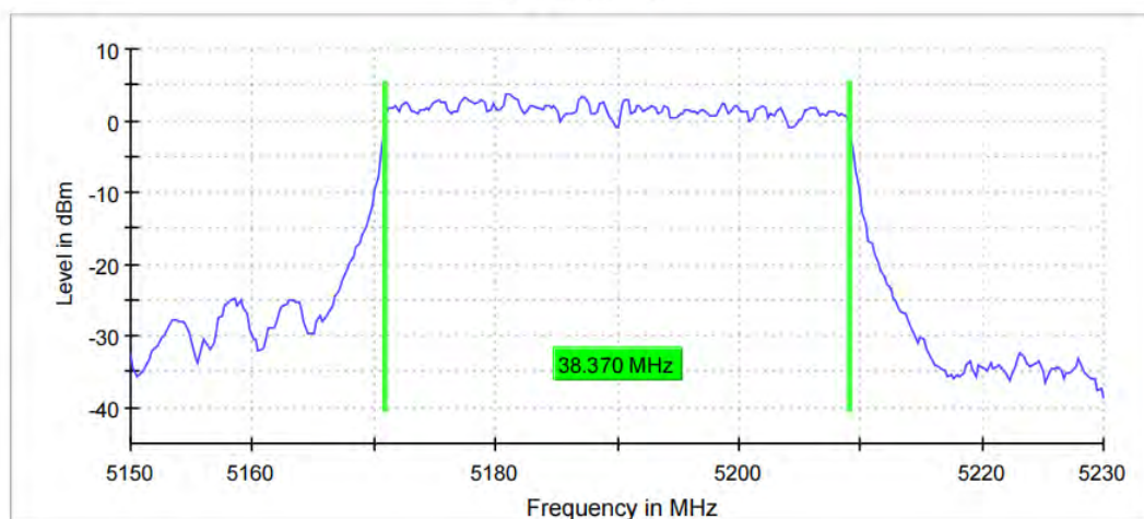
11AX40MIMO_Ant11_5190_484Tone_RU65 99 % Bandwidth
