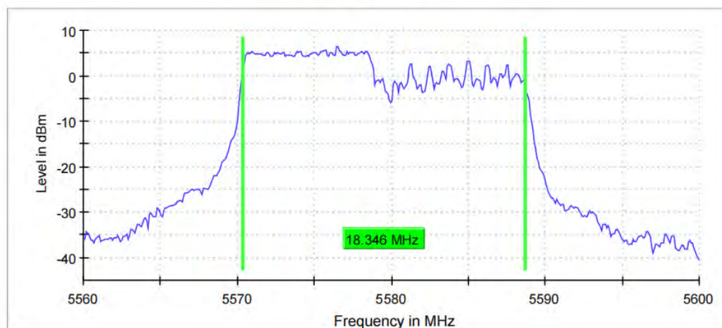
11AX20MIMO_Ant11_5580_242Tone_RU61
