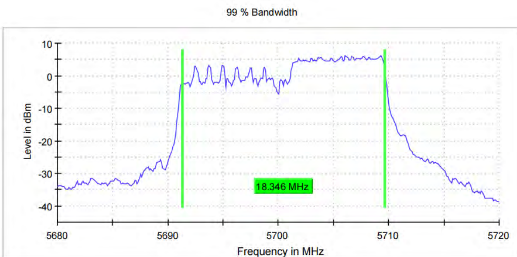
11AX20MIMO Ant11 5700 106Tone RU53
