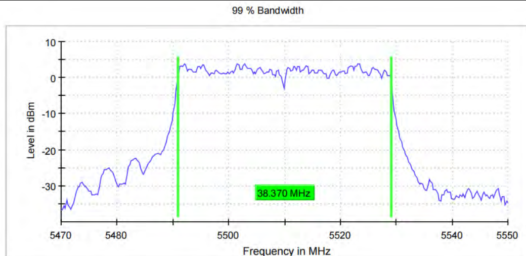
11AX40MIMO_Ant8_5510_484Tone_RU65
