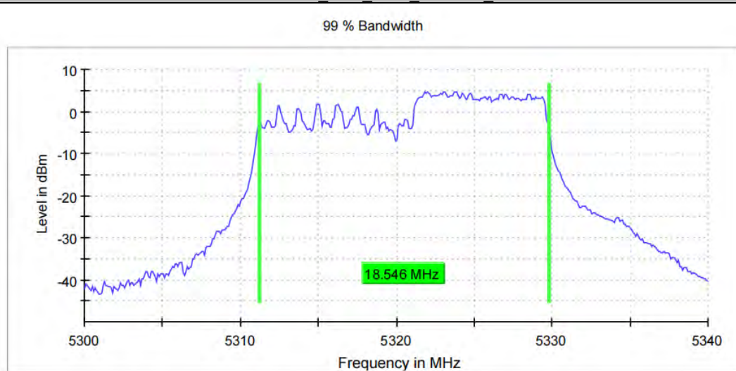
11AX20MIMO_Ant8_5320_106Tone_RU54
