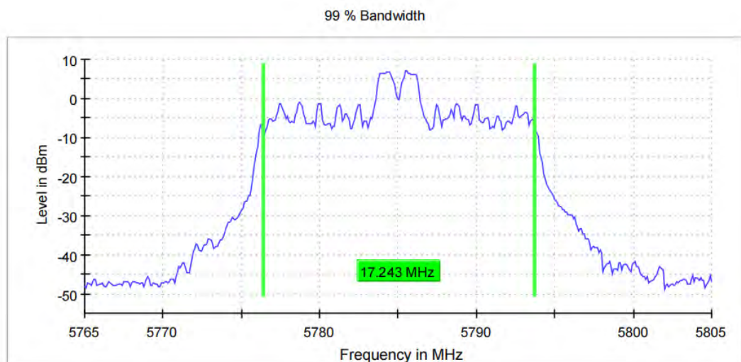
11AX20MIMO_Ant11_5785_26Tone_RU0
