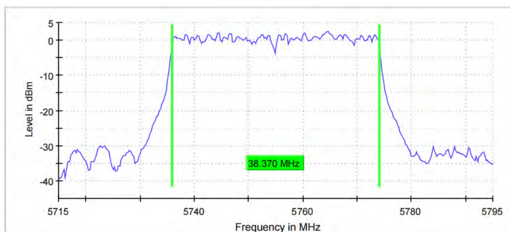
11AX40MIMO_Ant11_5755_484Tone_RU65
