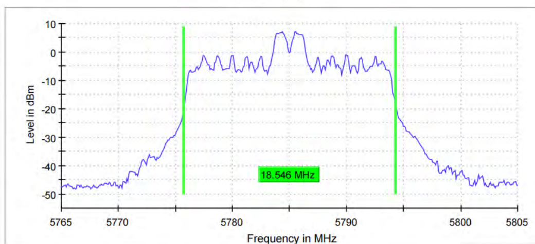
11AX20MIMO_Ant11_5785_52Tone_RU37
