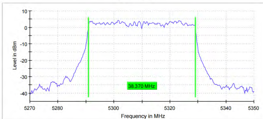
11AX40MIMO_Ant11_5310_484Tone_RU65
