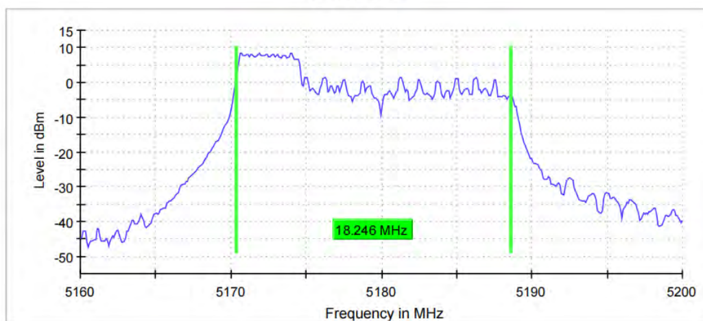
11AX20MIMO_Ant8_5180_106Tone_RU53
