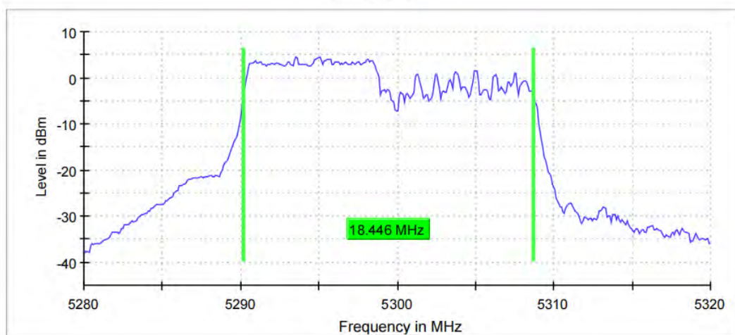
11AX20MIMO_Ant11_5300_242Tone_RU61
