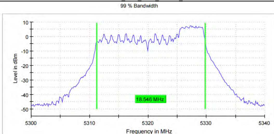
11AX20MIMO_Ant8_5320_52Tone_RU40
