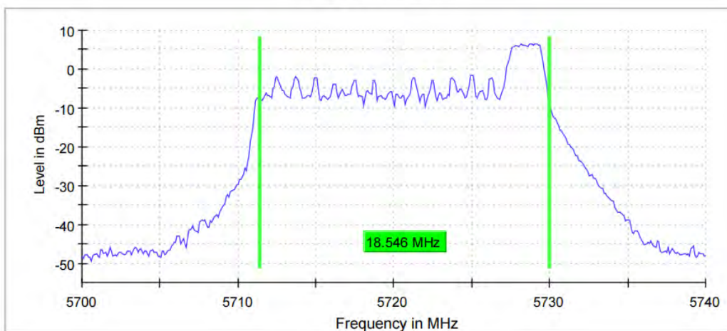
11AX20MIMO_Ant11_5720_52Tone_RU37
