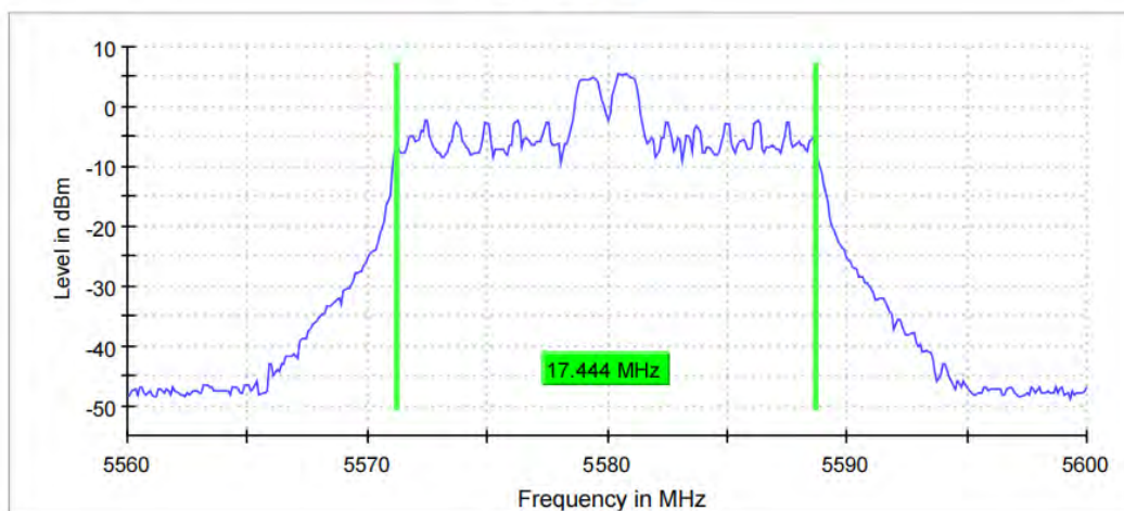
11AX20MIMO_Ant8_5580_52Tone_RU37
