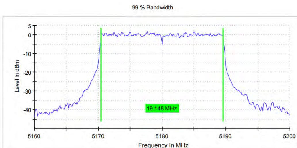
11AX20MIMO_Ant11_5180_242Tone_RU61
