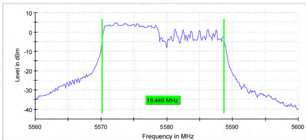
11AX20MIMO_Ant8_5580_106Tone_RU53
