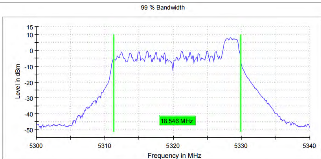
11AX20MIMO_Ant8_5320_52Tone_RU40
