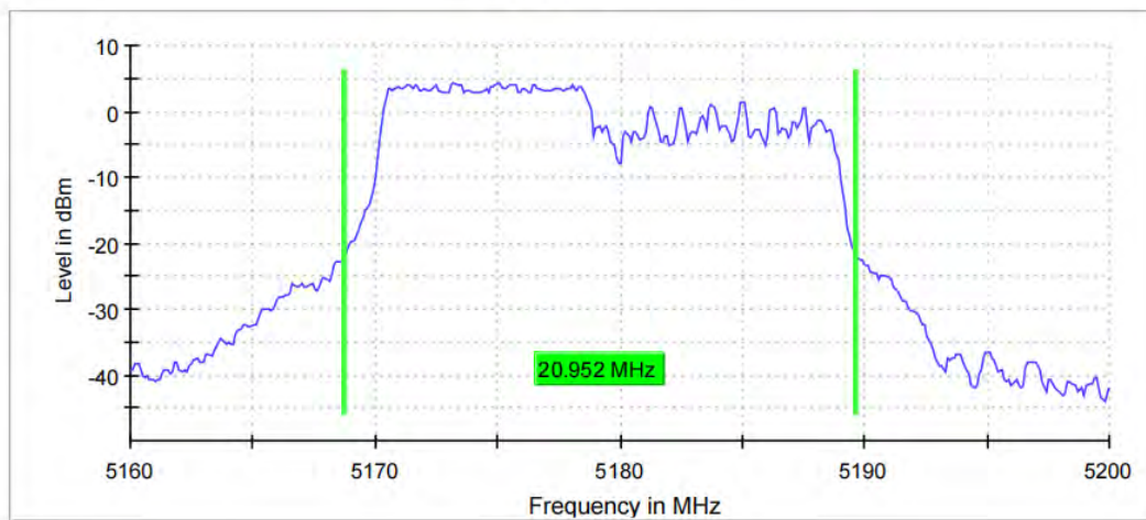
11AX20MIMO_Ant11_5180_242Tone_RU61
