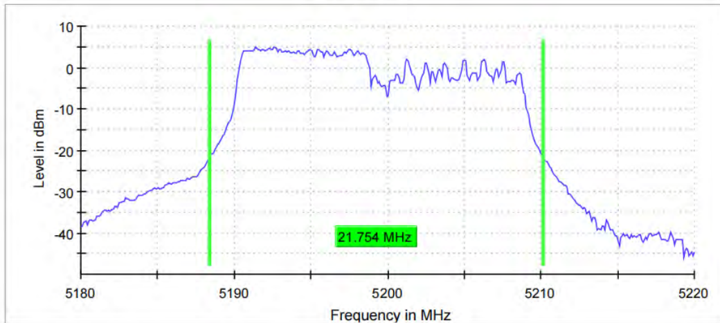
11AX20MIMO_Ant8_5200_106Tone_RU53
