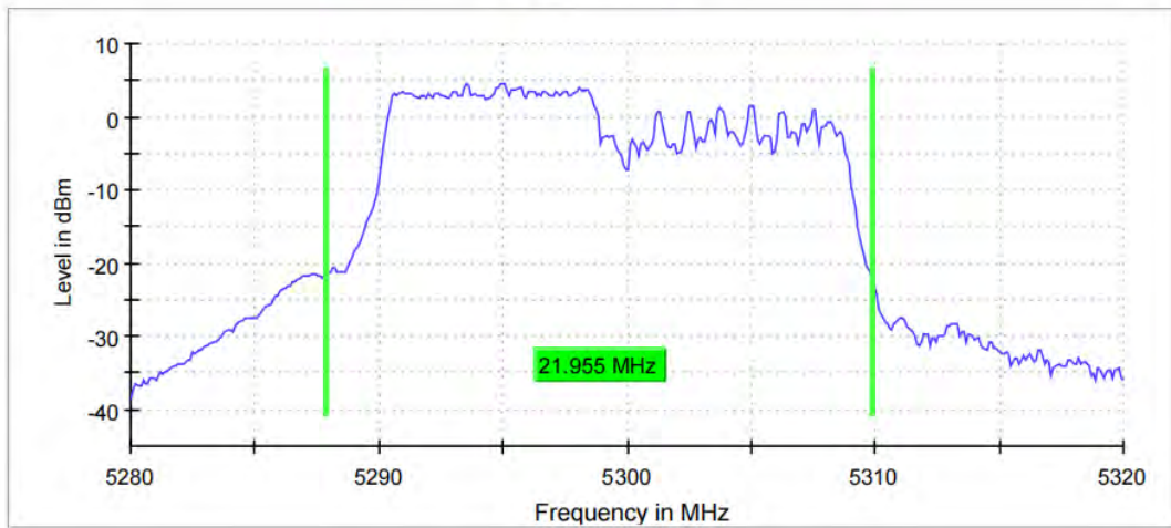
11AX20MIMO_Ant11_5300_242Tone_RU61
