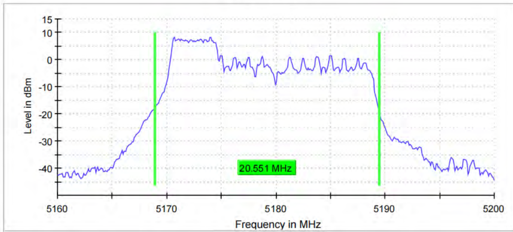
11AX20MIMO_Ant11_5180_106Tone_RU53
