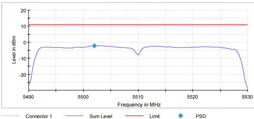
11N40_Ant11_5510
