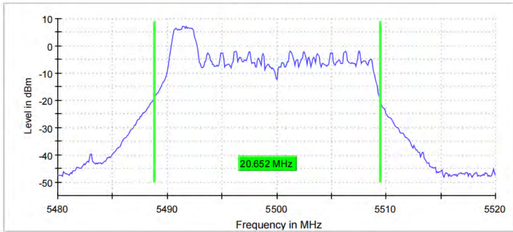
11AX20MIMO_Ant8_5500_52Tone_RU37
