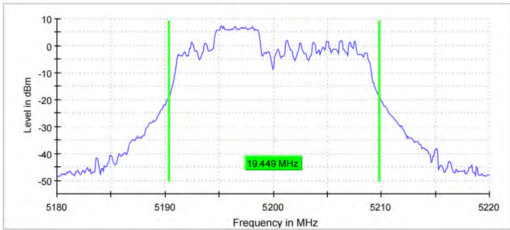
11AX20MIMO_Ant8_5200_106Tone_RU53
