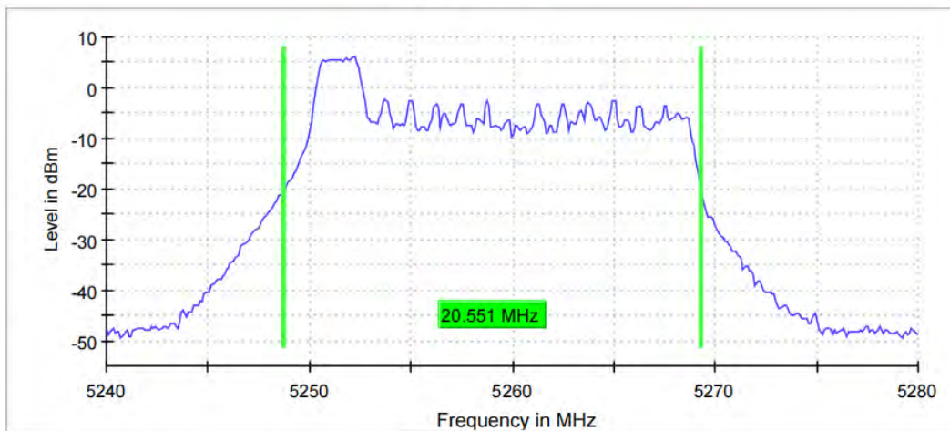
11AX20MIMO_Ant11_5260_52Tone_RU37
