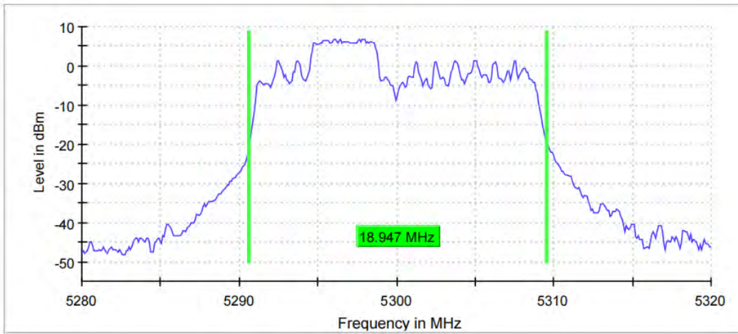
11AX20MIMO_Ant11_5300_106Tone_RU53
