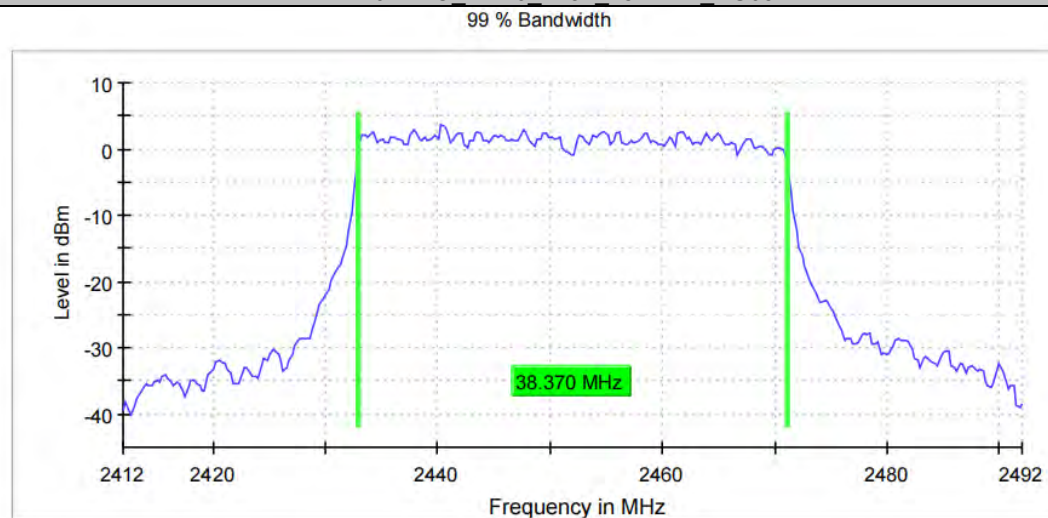
11AX40MIMO_Ant10_2452_484Tone_RU65
