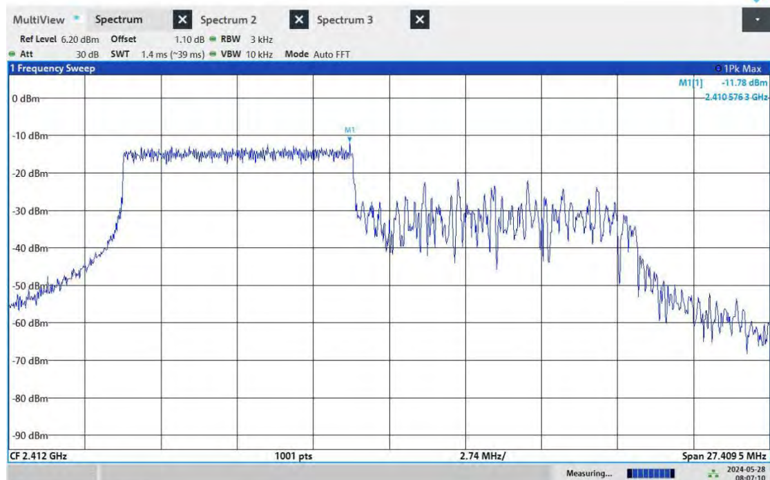
11AX20MIMO_Ant10_2412_242Tone_RU61
