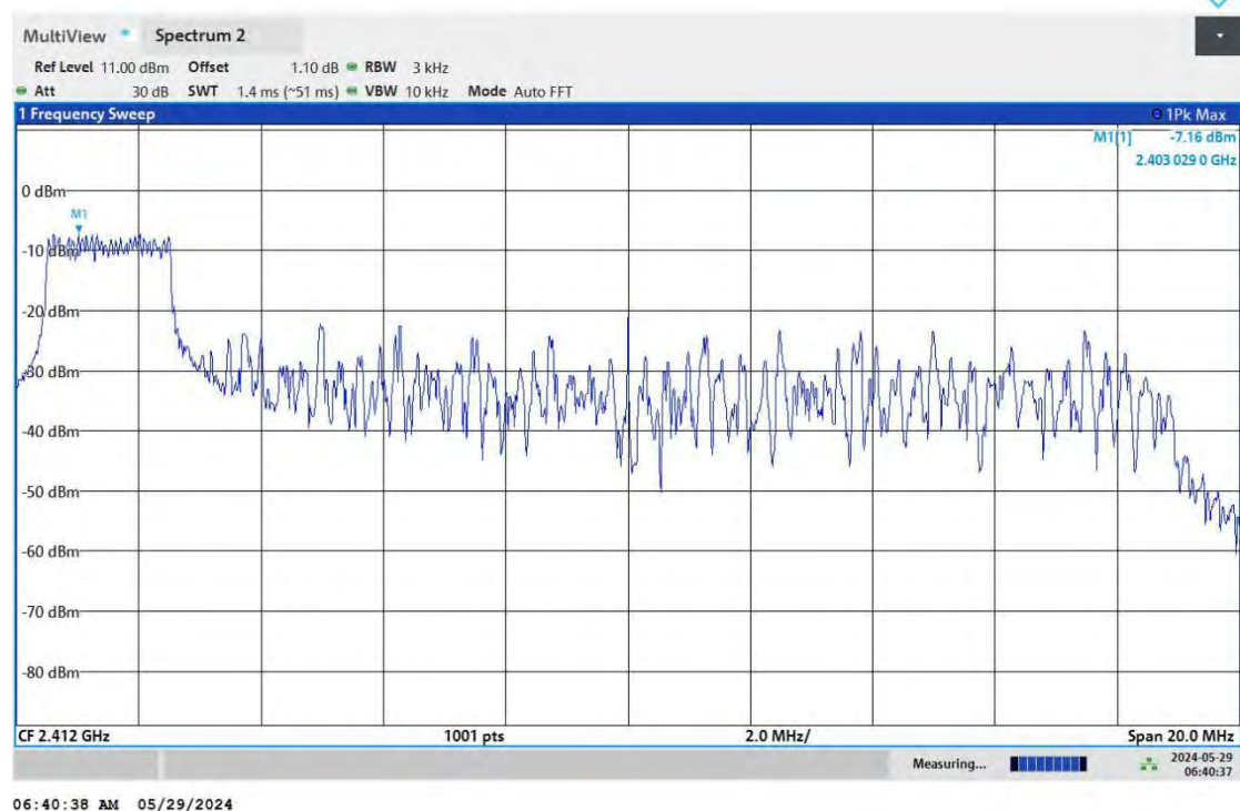
11AX20MIMO_Ant9_2412_52Tone_RU37
