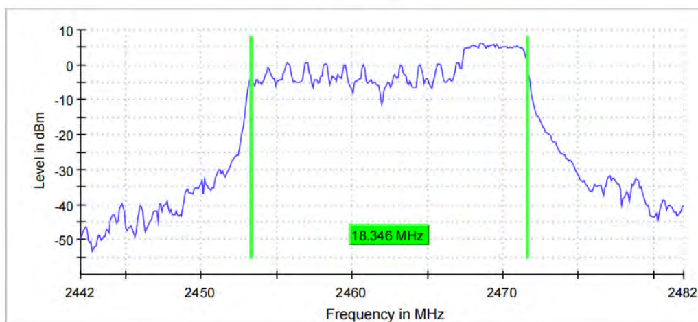
11AX20MIMO_Ant10_2462_106Tone_RU54
