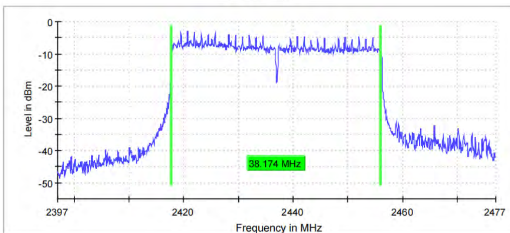
11AX40MIMO_Ant10_2437_484Tone_RU65
