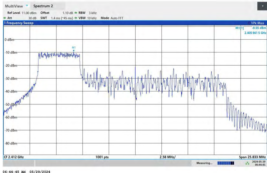
11AX20MIMO_Ant9_2412_106Tone_RU53
