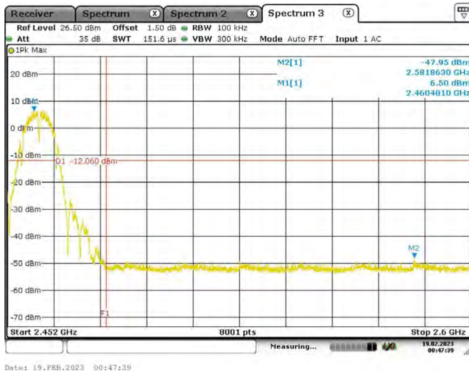
11B_Ant0_High_2462
