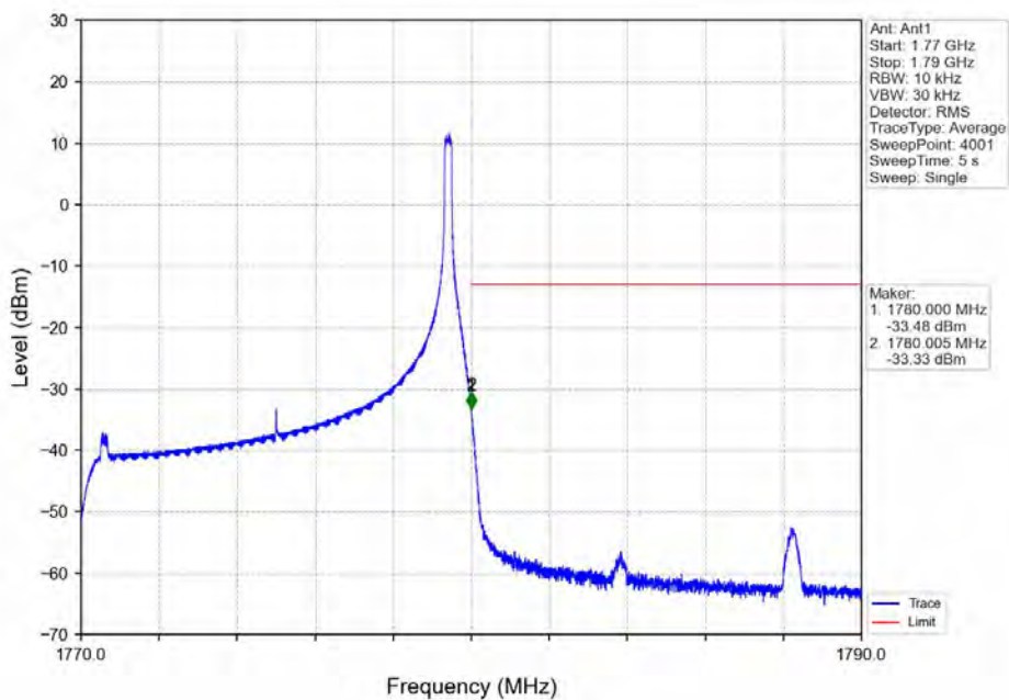
Band66_10MHz_QPSK_HCH_1775MHz_RB_1_49_NTNV
