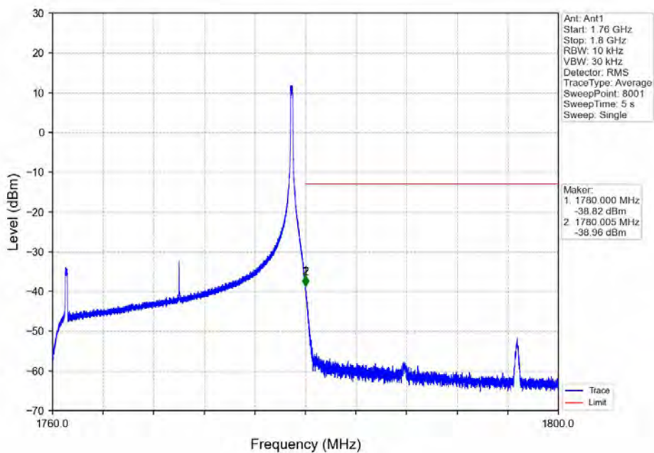
Band66_20MHz_QPSK_HCH_1770MHz_RB_1_99_NTNV
