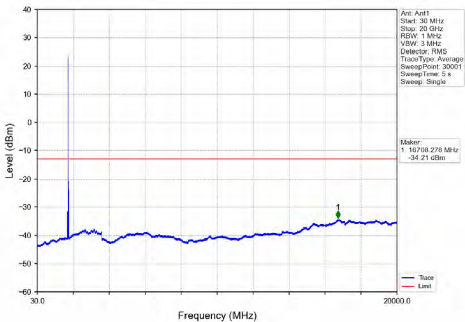
Band66_20MHz_QPSK_MCH_1745MHz_RB_1_0_NTNV
