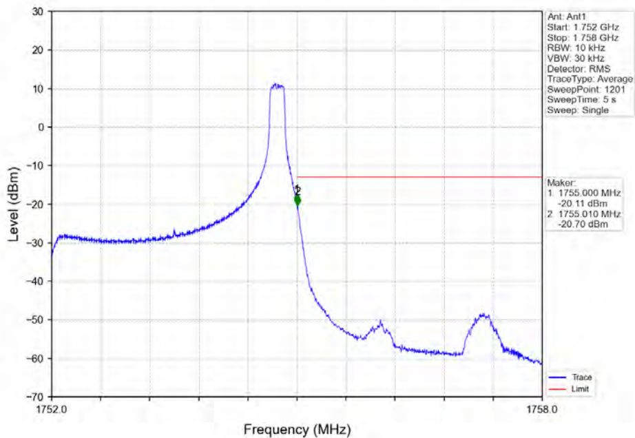
Band4_3MHz_QPSK_HCH_1753.5MHz_RB_1_14_NTNV
