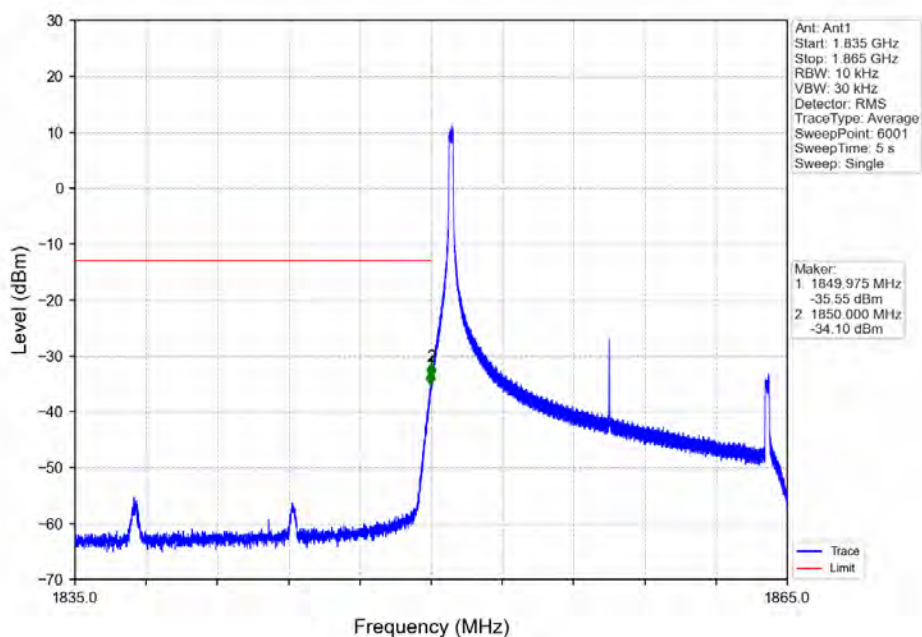
Band2 15MHz 64QAM LCH 1857.5MHz RB 1 0 NTNV
