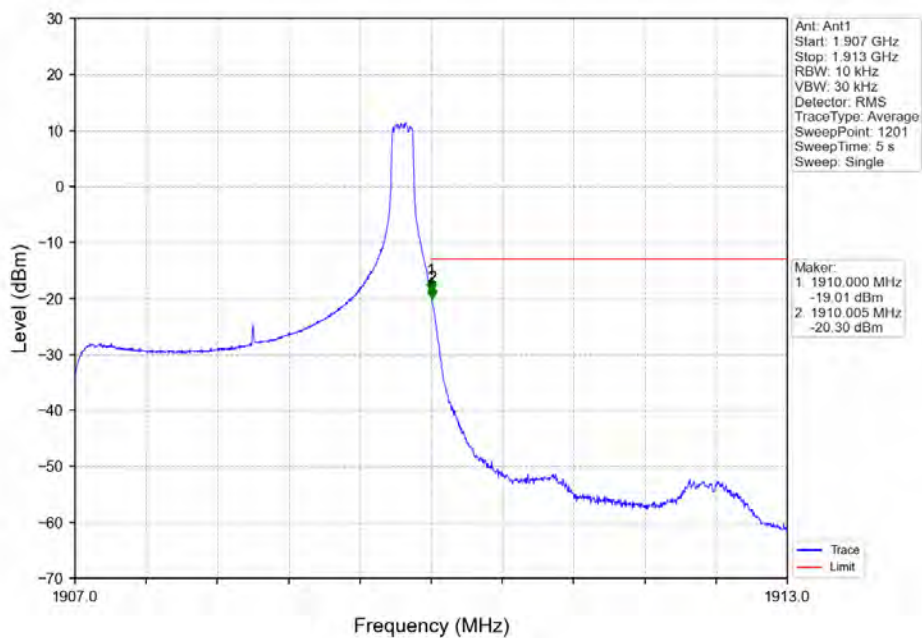
Band2_3MHz_QPSK_HCH_1908.5MHz_RB_1_14_NTNV
