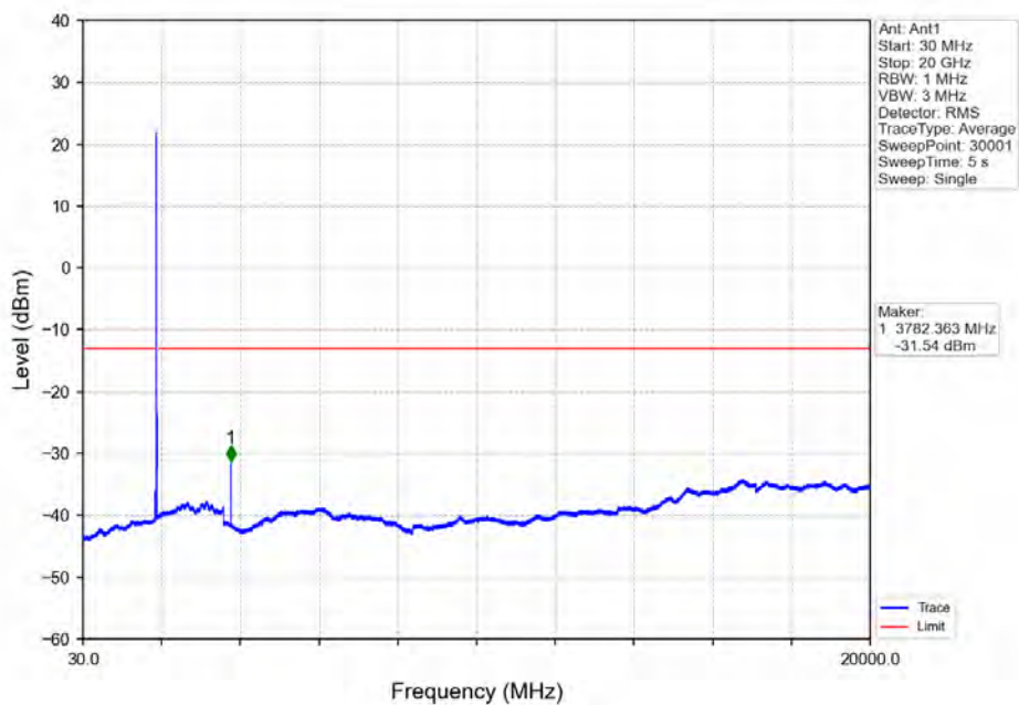
Band2_20MHz_16QAM_HCH_1900MHz_RB_1_0_NTNV
