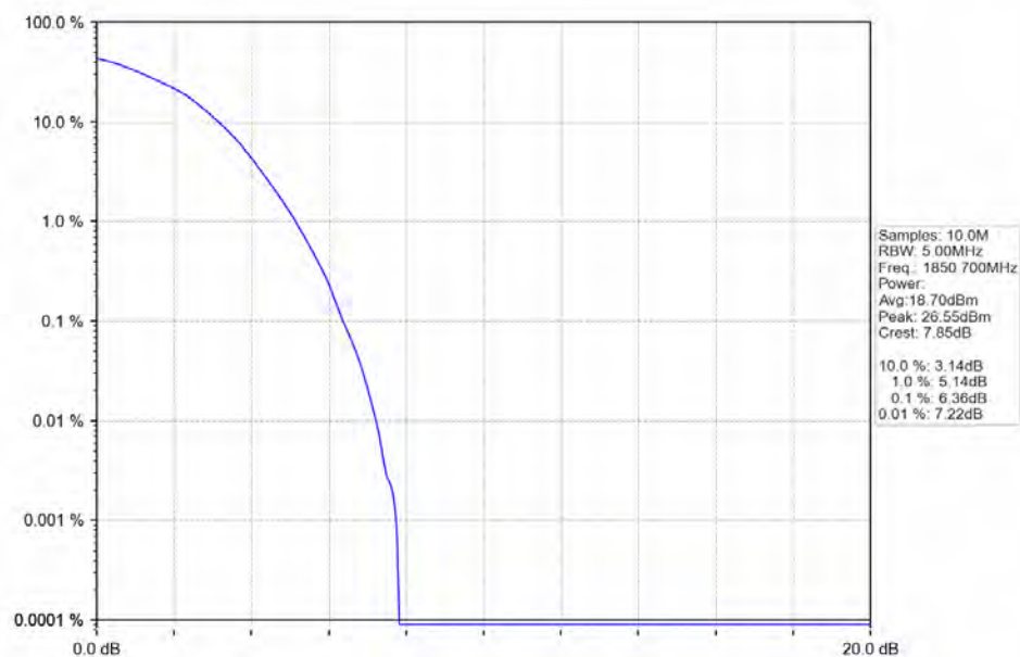
Band2 1.4MHz 64QAM LCH 1850.7MHz RB 6 0 NTV
