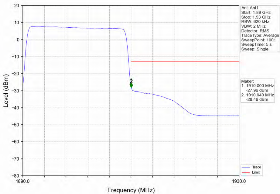
Band2_20MHz_16QAM_HCH_1900MHz_RB_100_0_NTNV
