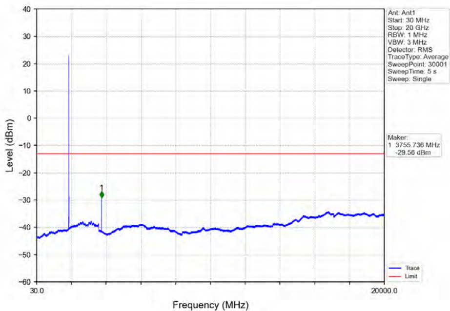
Band2_5MHz_QPSK_MCH_1880MHz_RB_1_0_NTNV
