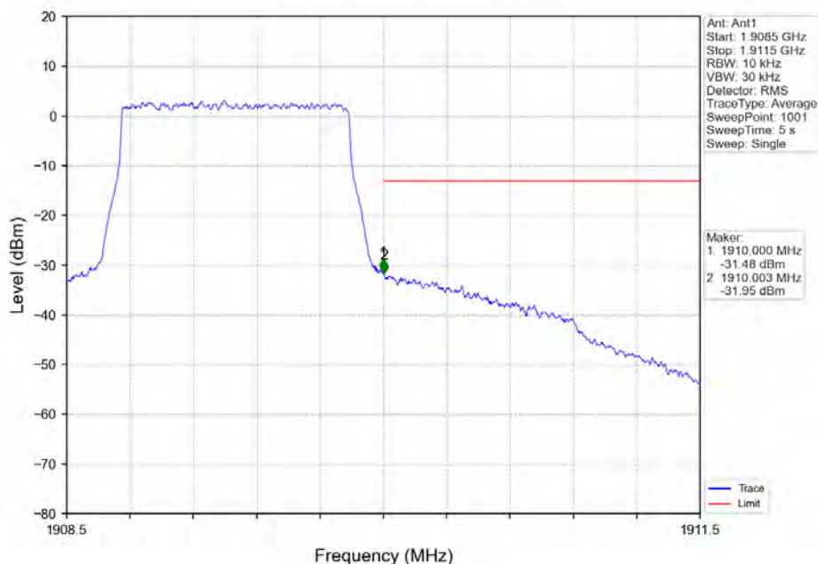
Band2 1.4MHz 64QAM HCH 1909.3MHz RB 1 5 NTNV
