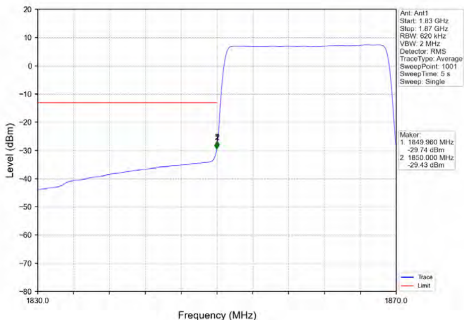
Band2_20MHz_16QAM_LCH_1860MHz_RB_100_0_NTNV
