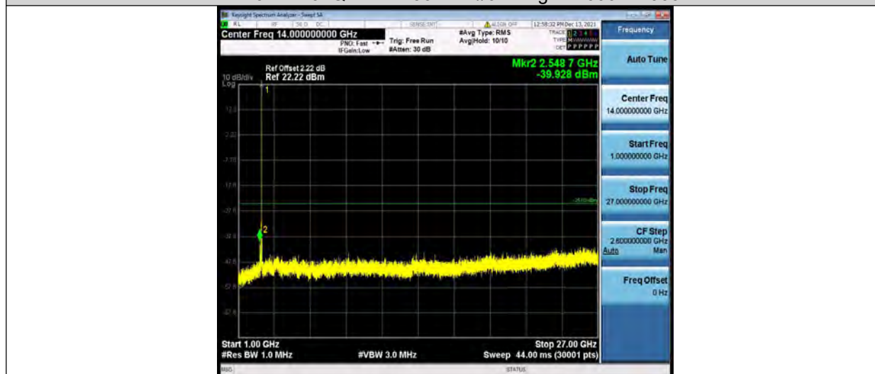
Band41-20MHz-64QAM-41490-1RB#0-Range2:1000~27000MHz
