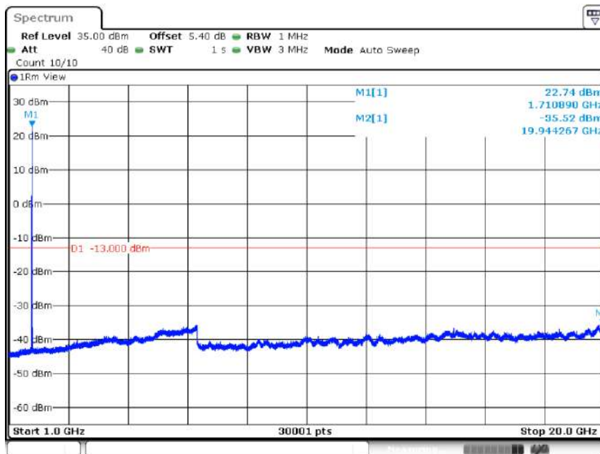
Band4-20MHz-QPSK-20050-1RB#0-Range2:1000~20000MHz
