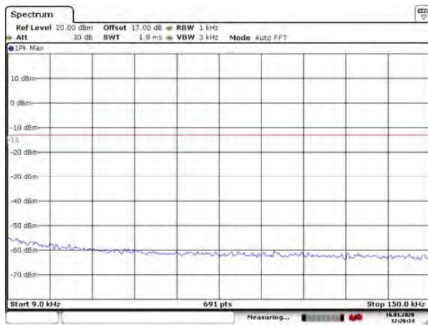
GSM 1900 CH-Low 9kHz ~ 150kHz
