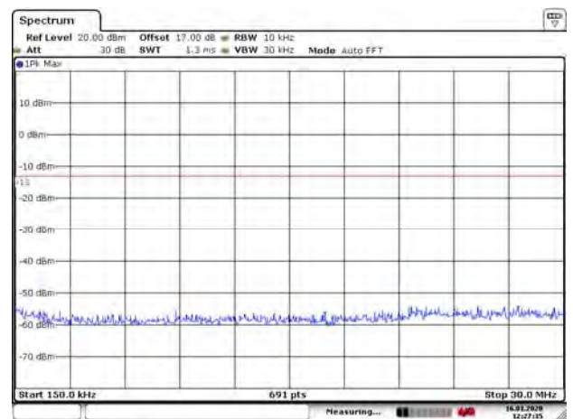
GSM 1900 CH- Middle 150kHz ~ 30MHz
