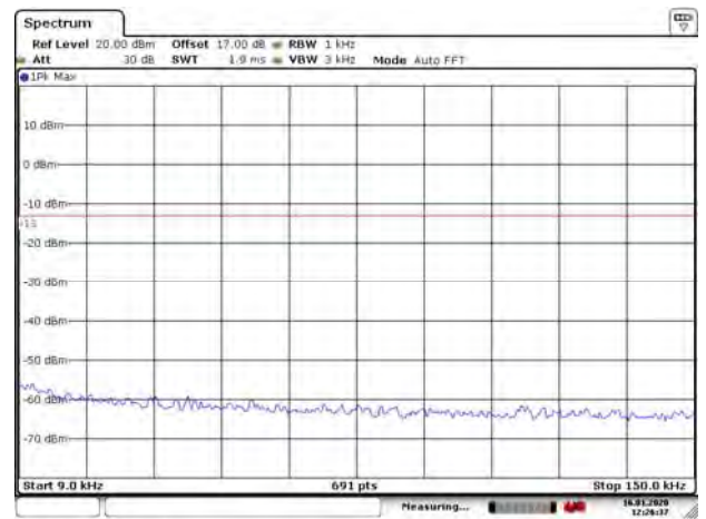
GSM 1900 CH- Middle 9kHz ~ 150kHz
