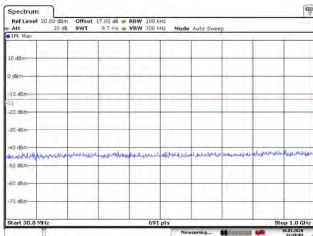
GSM 1900 CH-Low 30MHz ~ 1GHz
