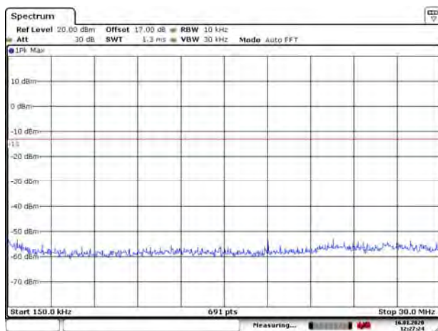
GSM 1900 CH-Low 150kHz ~ 30MHz
