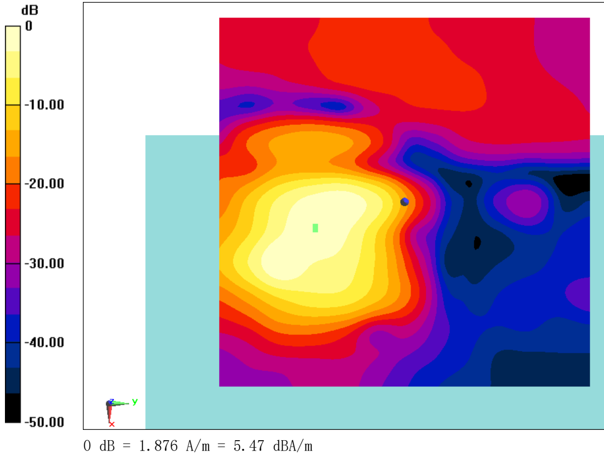
Fig B.24 T-Coil EDGE 850
