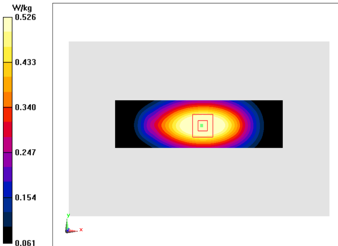
Fig.6 WCDMA 850
