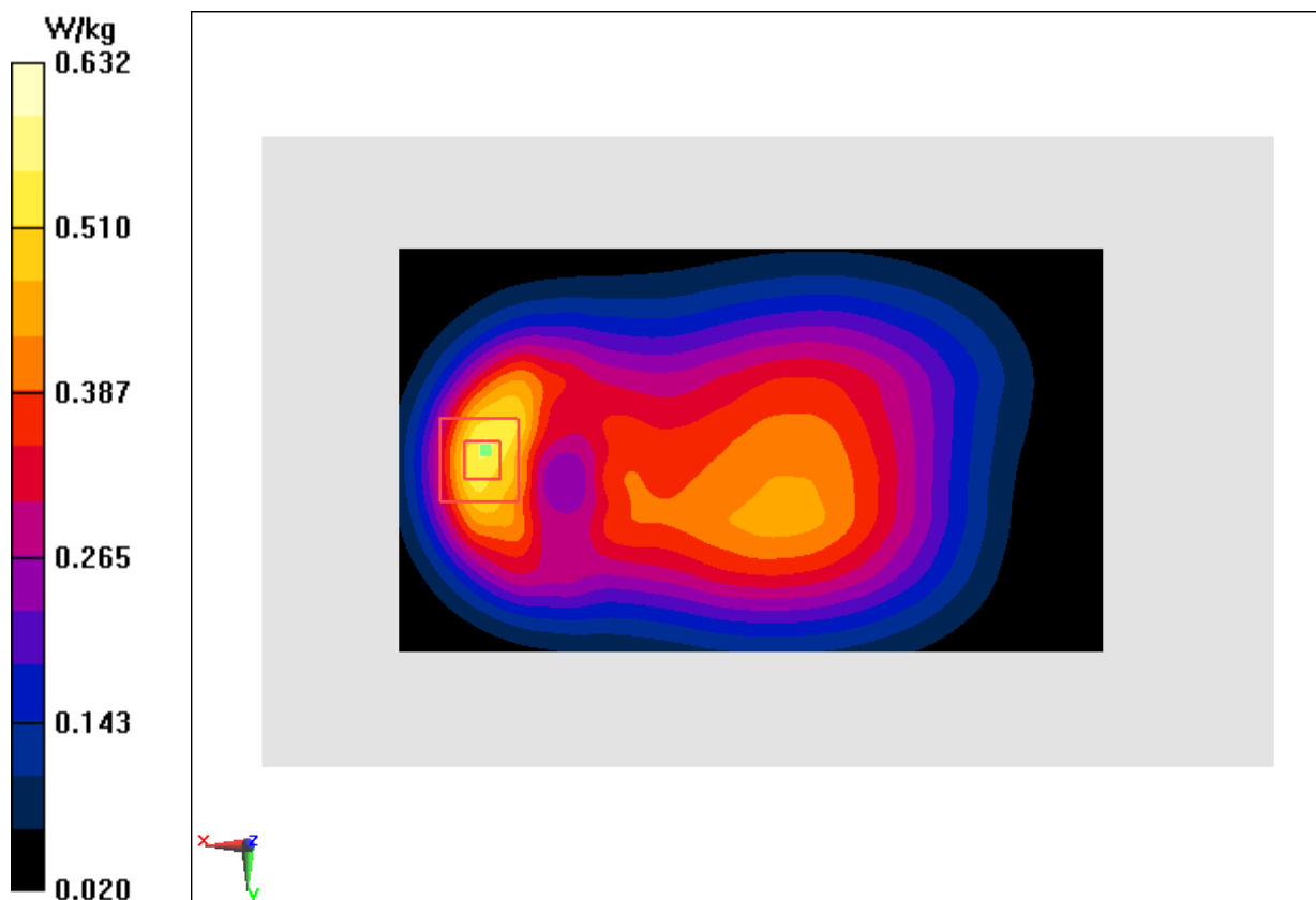
Fig.8LTE Band5
