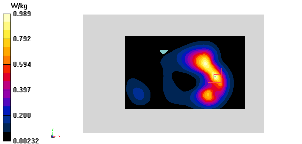
Fig.10 LTE Band7
