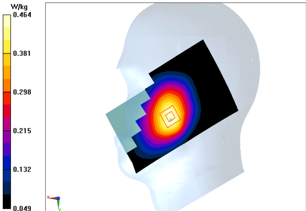
Fig.5 WCDMA 850
