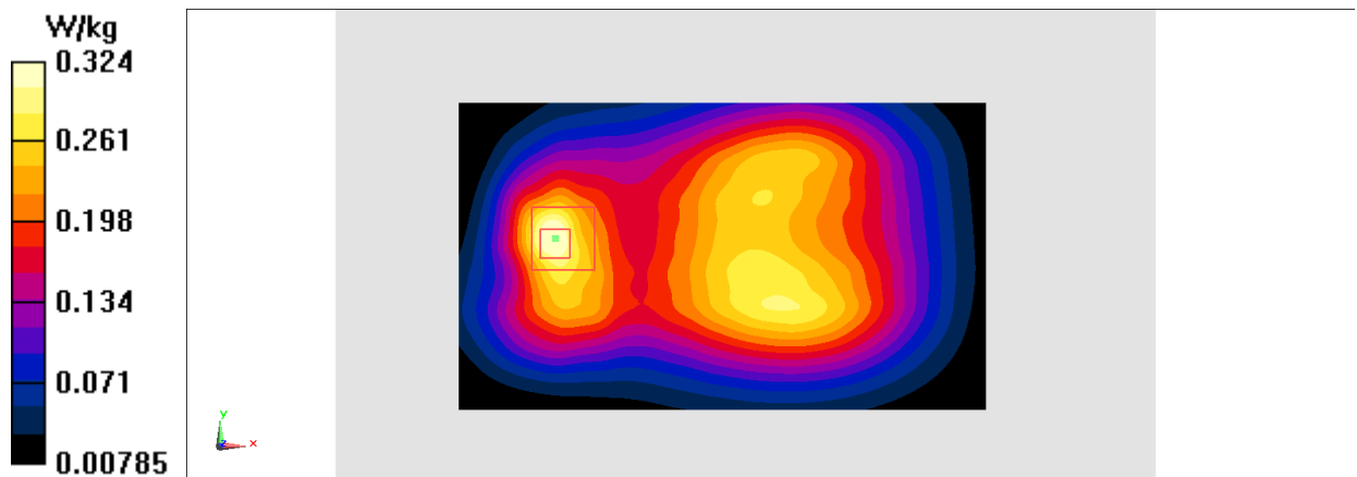
Fig.6 WCDMA 850
