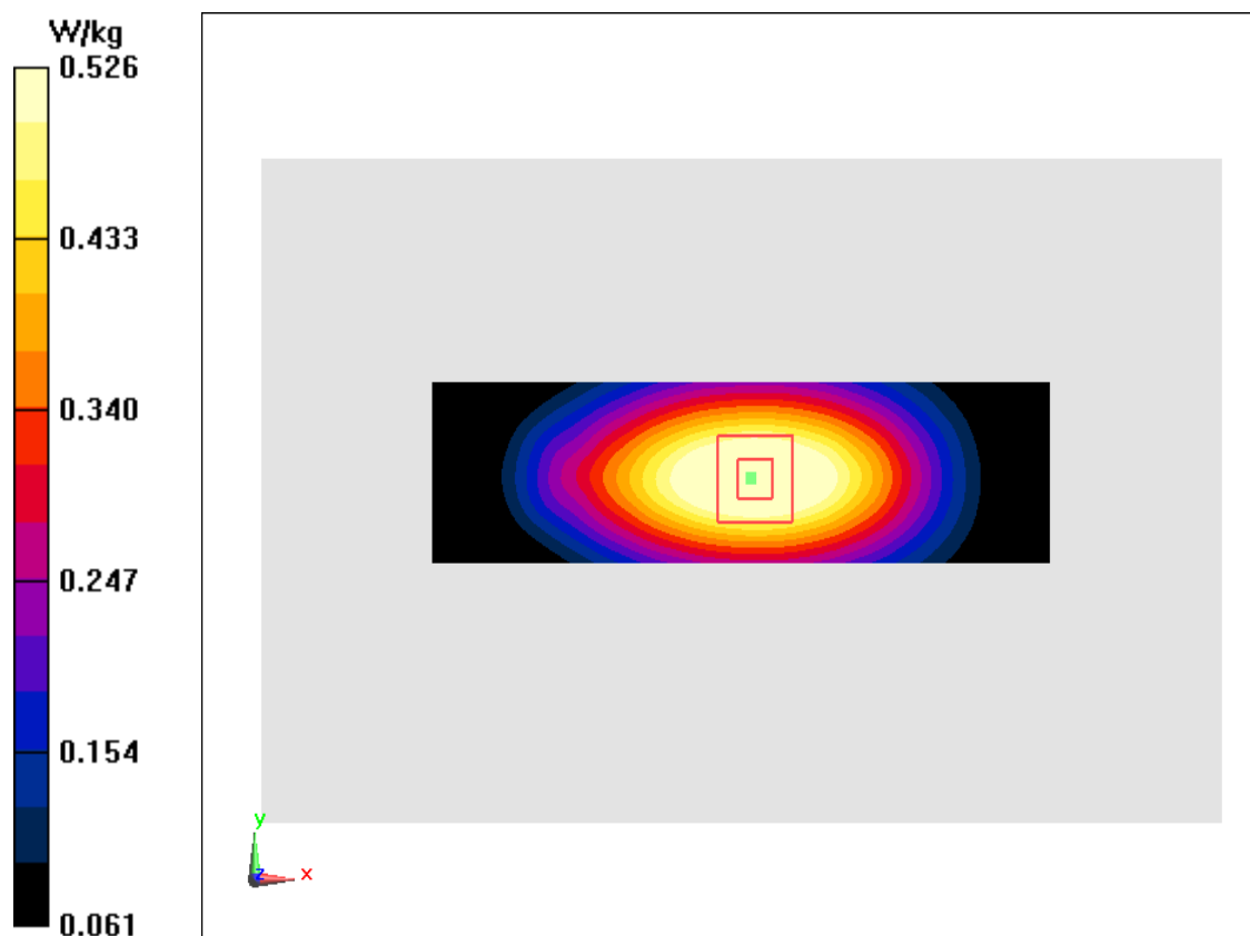
Fig.6 WCDMA 850
