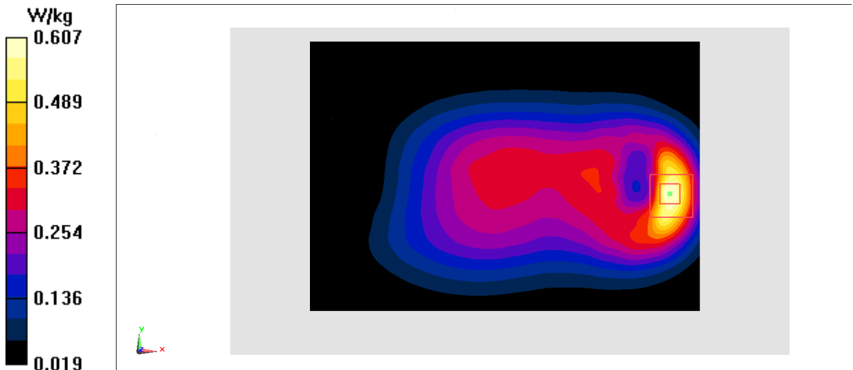
Fig.14 LTE Band5
