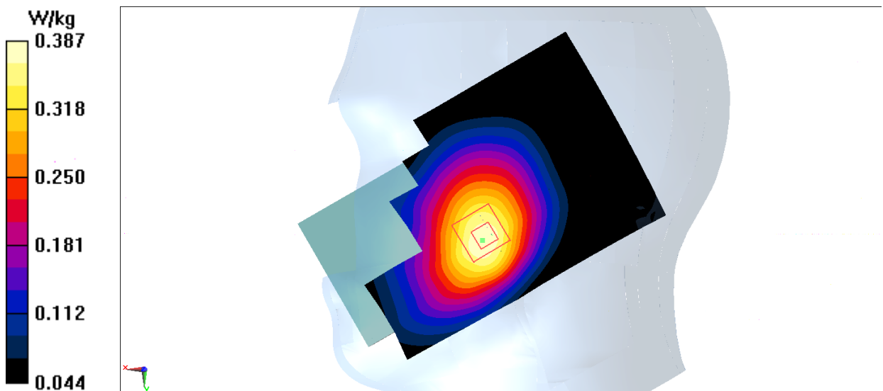
Fig.5 WCDMA 850
