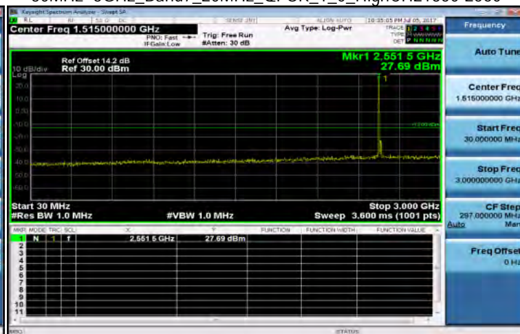
30MHz~3GHz_Band7_20MHz_QPSK_1_0_HighCH21350-2560
